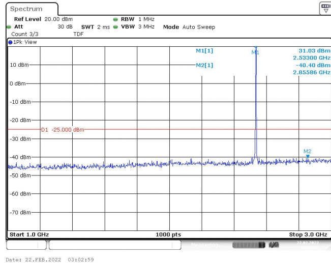
Band7-5MHz-QPSK-21100-1RB#0-Range2:1000~3000MHz
