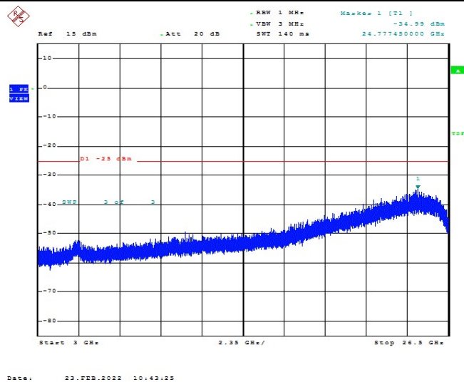
Band7-5MHz-QPSK-21425-1RB#0-Range1:3000~26500MHz
