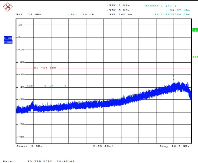
Band7-5MHz-QPSK-21100-1RB#0-Range1:3000~26500MHz
