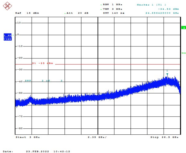
Band7-5MHz-QPSK-20775-1RB#0-Range1:3000~26500MHz
