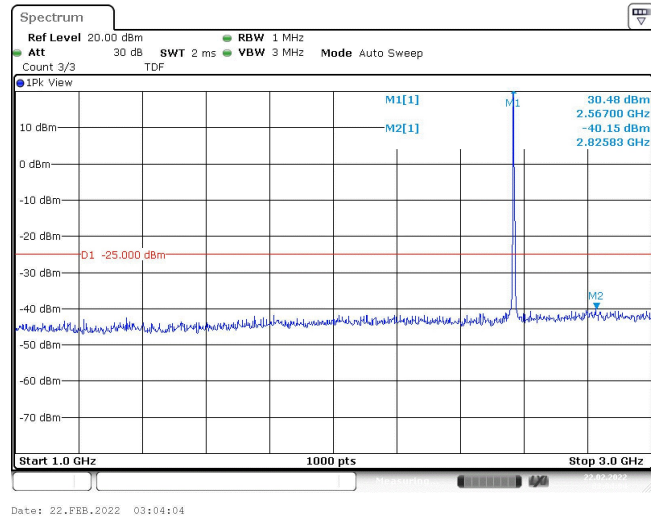
Band7-5MHz-QPSK-21425-1RB#0-Range2:1000~3000MHz
