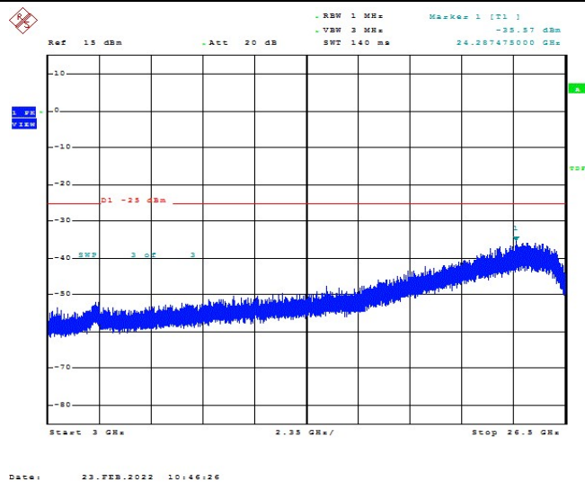
Band7-10MHz-QPSK-21100-1RB#0-Range1:3000~26500MHz
