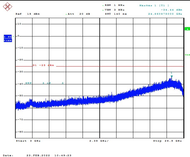
Band7-15MHz-QPSK-20825-1RB#0-Range1:3000~26500MHz
