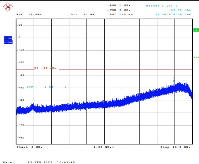
Band7-10MHz-QPSK-20800-1RB#0-Range1:3000~26500MHz
