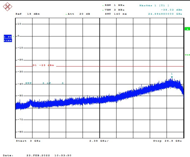
Band7-20MHz-QPSK-21350-1RB#0-Range1:3000~26500MHz
