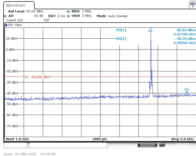
Band7-20MHz-QPSK-21100-1RB#0-Range2:1000~3000MHz
