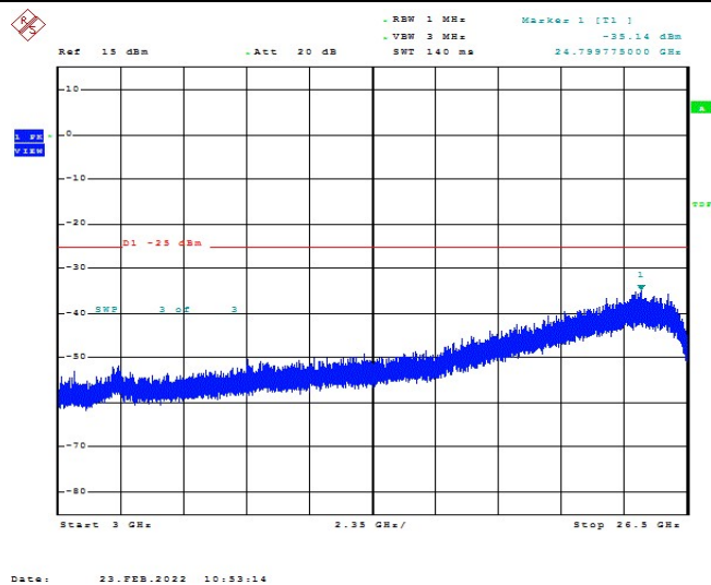
Band7-20MHz-QPSK-21100-1RB#0-Range1:3000~26500MHz
