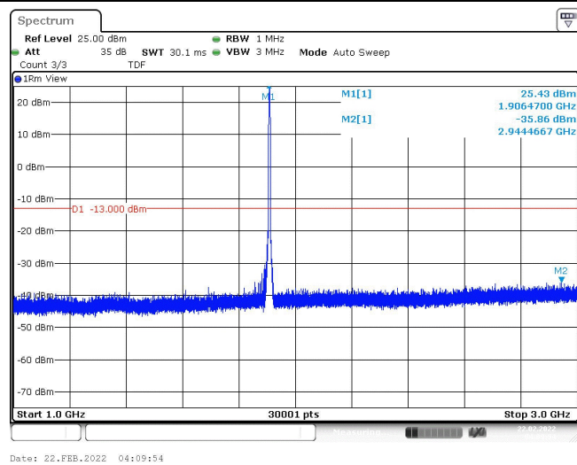
Band2-9538-4-1000~3000MHz
