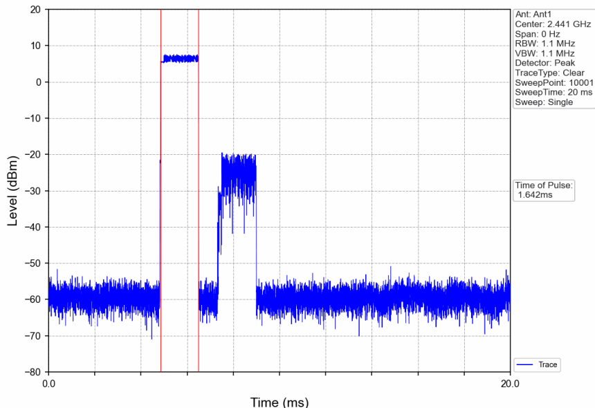
Pi/4DQPSK_2DH3_HOPP_Ant1_NTNV
