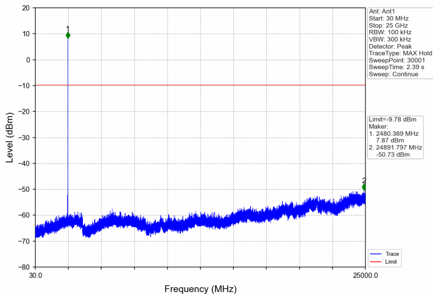
GFSK_DH5_HOPP_Ant1_NTNV
