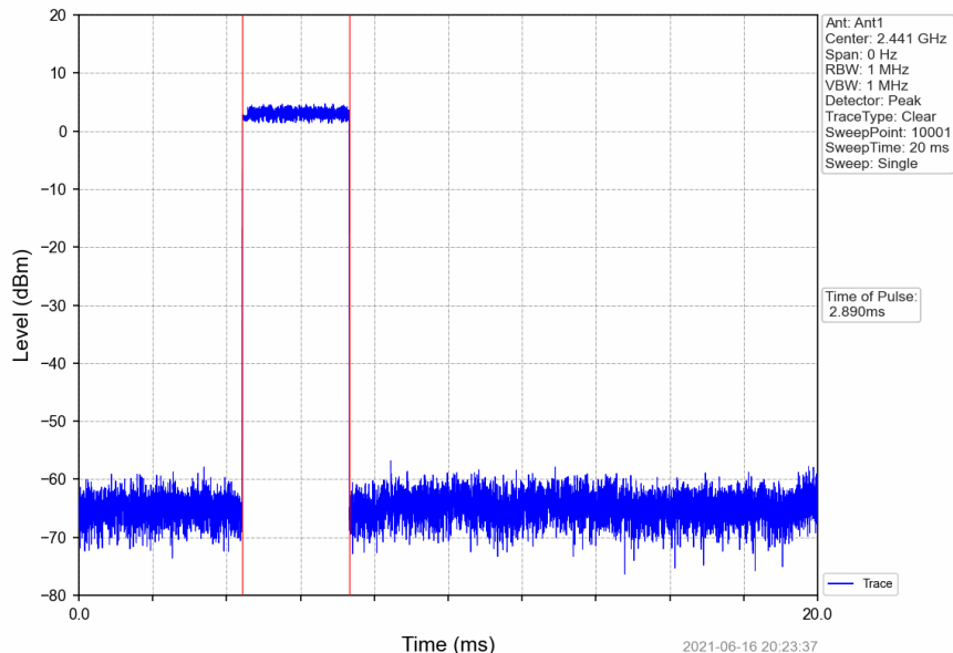
Pi/4DQPSK_2DH5_HOPP_Ant1_NTNV
