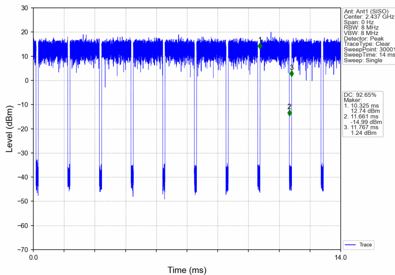
802.11n(HT20)_MCH_2437MHz_Ant1 (SISO)_NTNV
