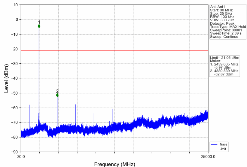
2M_MCH_2440MHz_Ant1 NTN
