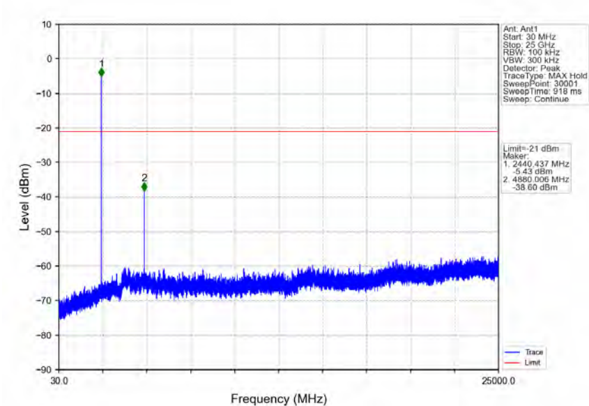
2M_MCH_2440MHz_Ant1_NTNV
