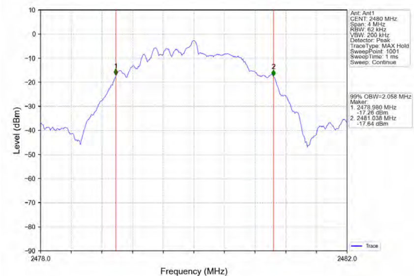
2M_HCH_2480MHz_Ant1_NTNV
