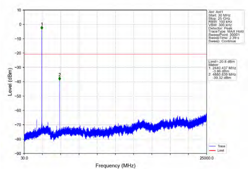
2M_MCH_2440MHz_Ant1_NTNV
