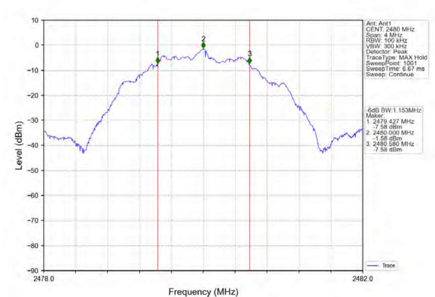
2M_HCH_2480MHz_Ant1_NTNV
