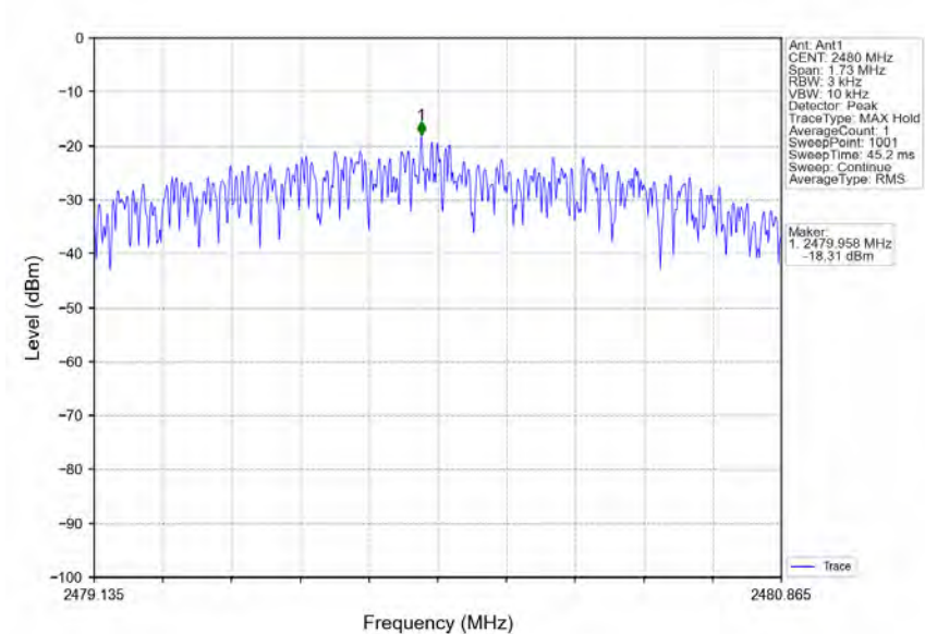
2M_HCH_2480MHz_Ant1_NTNV
