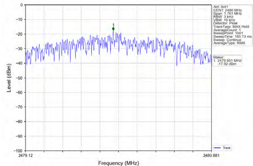
2M_HCH_2480MHz_Ant1_NTNV
