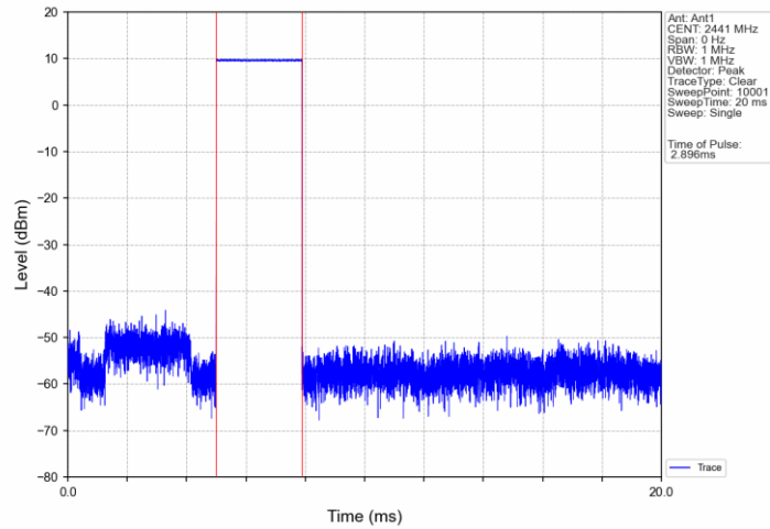
GFSK_DH5_HOPP_Ant1_NTNV
