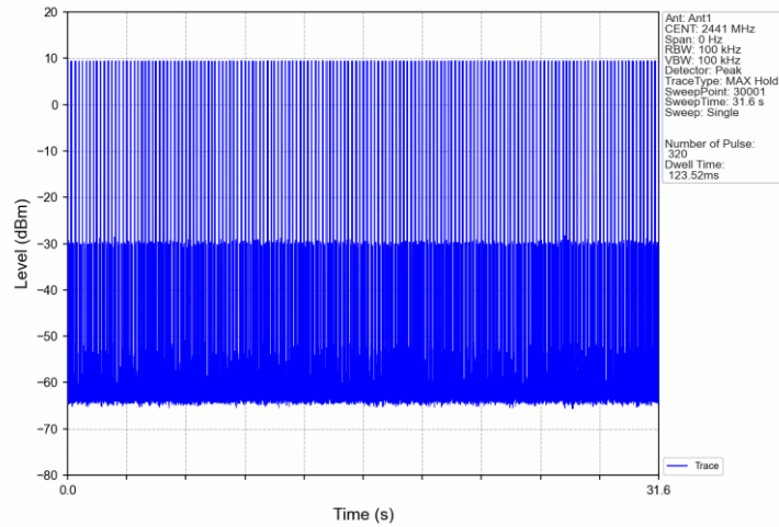
GFSK_DH3_HOPP_Ant1_NTNV
