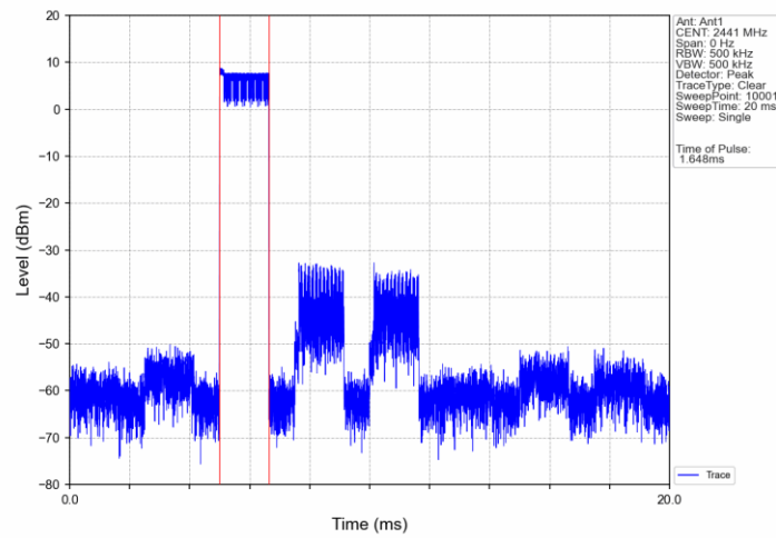
Pi/4DQPSK_2DH3_HOPP_Ant1_NTNV
