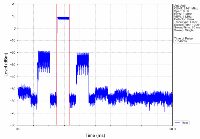
8DPSK_3DH3_HOPP_Ant1_NTNV
