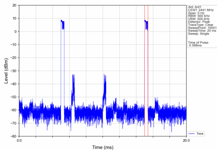
Pi/4DQPSK_2DH1_HOPP_Ant1_NTNV
