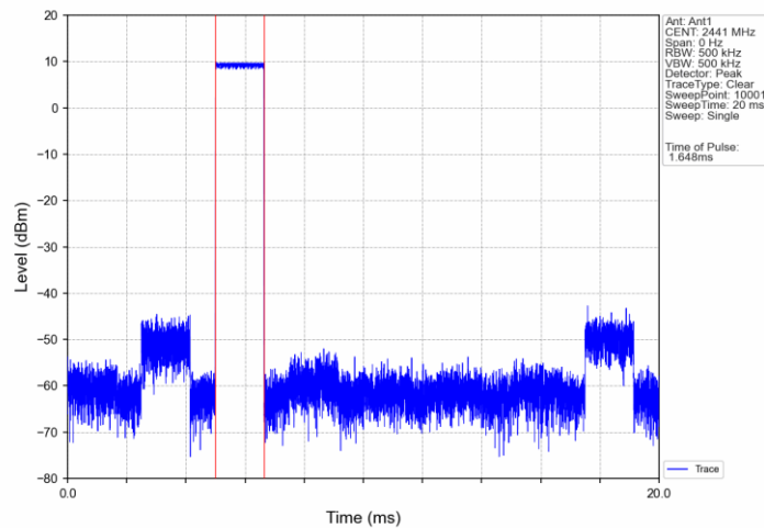
GFSK_DH3_HOPP_Ant1_NTNV
