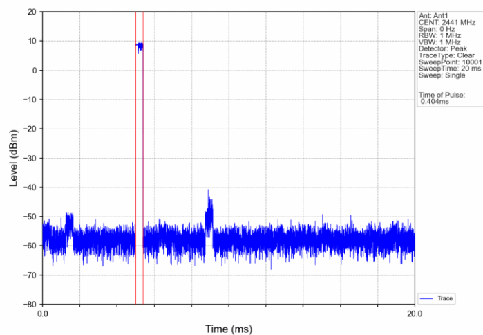
8DPSK_3DH1_HOPP_Ant1_NTNV
