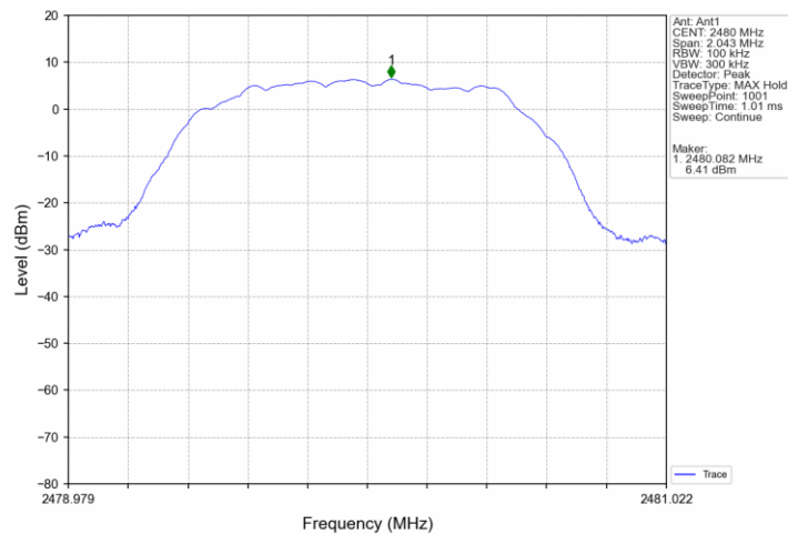
8DPSK 3DH5 HOPP Ant1 NTNv
