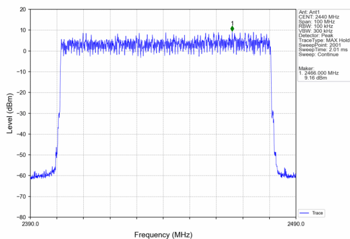
8DPSK 3DH5 HOPP Ant1 NTNv
