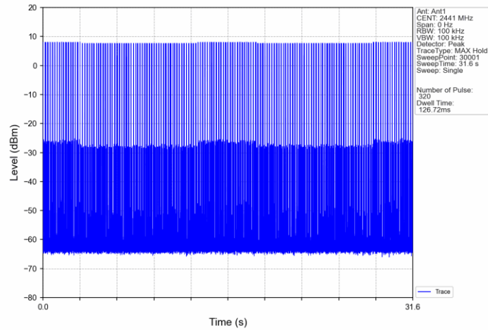
8DPSK 3DH3_HOPP_Ant1_NTNV
