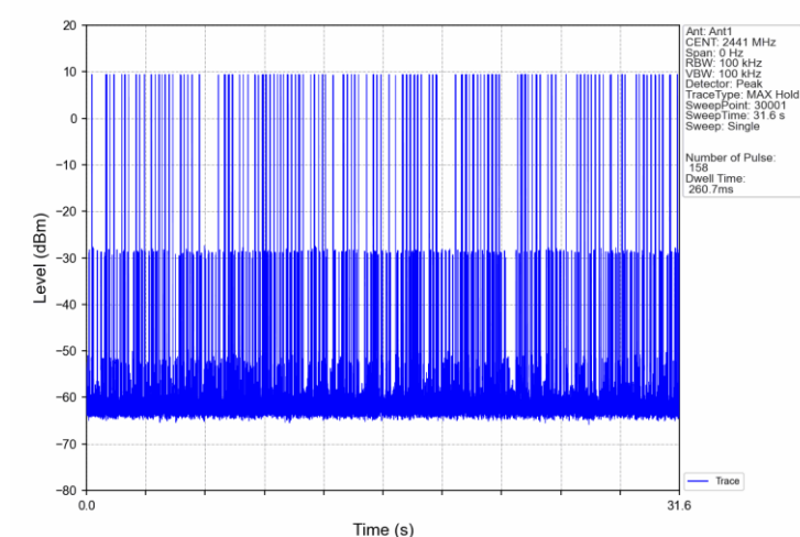
GFSK_DH5_HOPP_Ant1_NTNV
