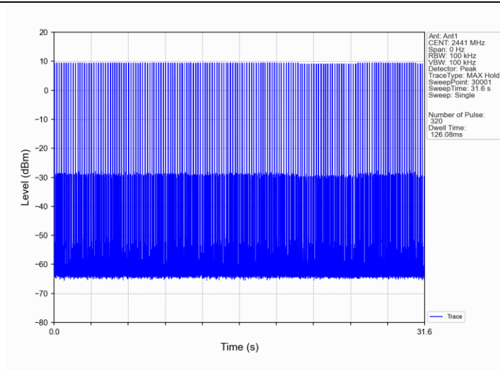
GFSK_DH3_HOPP_Ant1_NTNV
