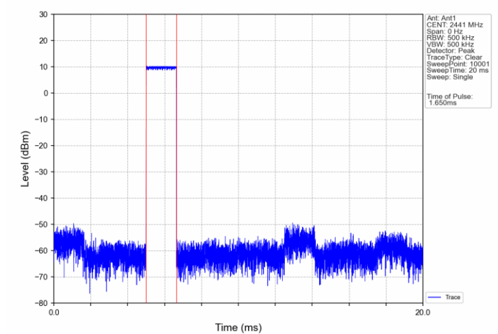
GFSK_DH3_HOPP_Ant1_NTNV
