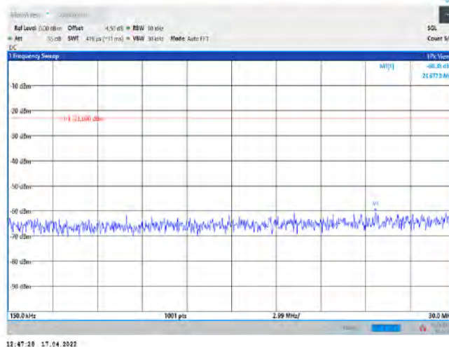
Band26-10MHz-QPSK-26740-1RB#0-Range2:0.15~30MHz
