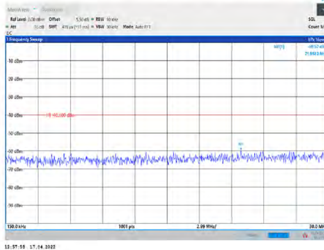
Band30-10MHz-QPSK-27710-1RB#0-Range2:0.15~30MHz
