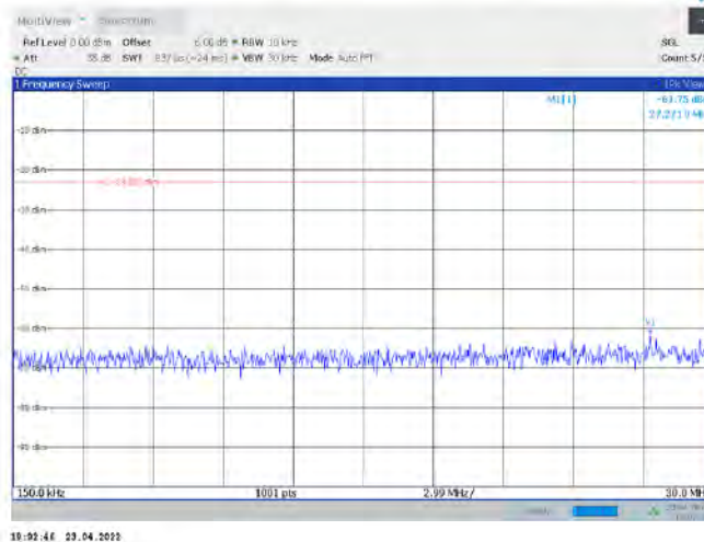
Band42-20MHz-QPSK-42190-1RB#0-Range2:0.15~30MHz
