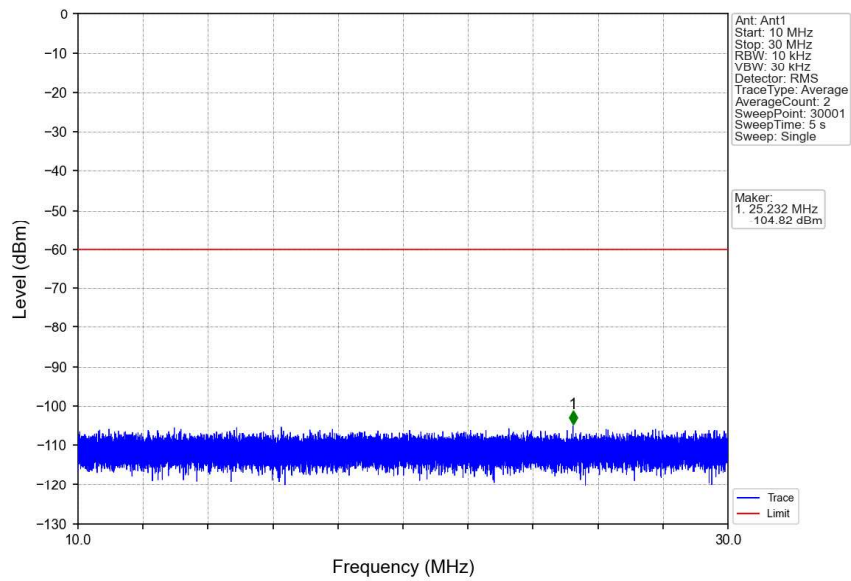
n48_30kHz_SISO_NTNV_10MHz_DFT-s-OFDM QPSK_3555MHz_Edge_1RB_Left
