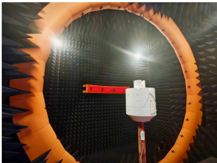
探头微波暗室
