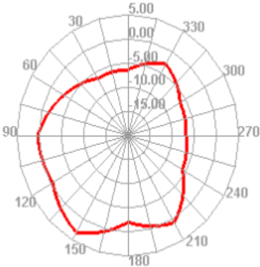
2500.000MHz E2
