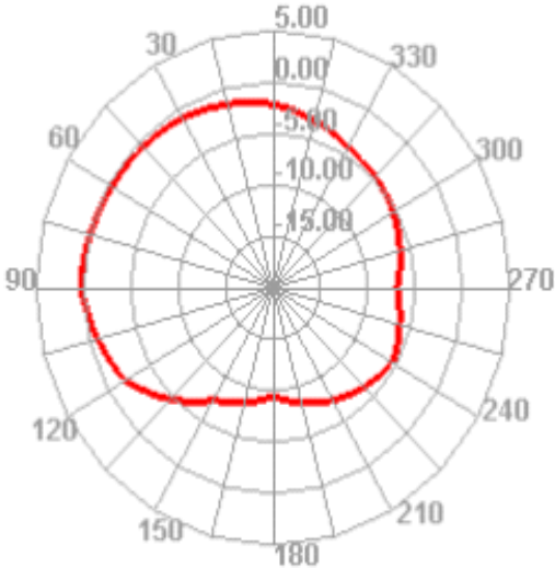
2500.000MHz H
