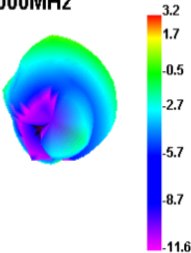
2500.000MHz
