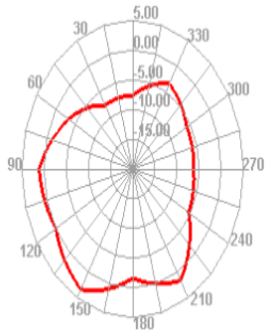
2450.000MHz E2
