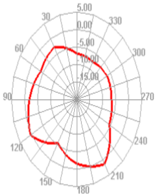
2450.000MHz E1
