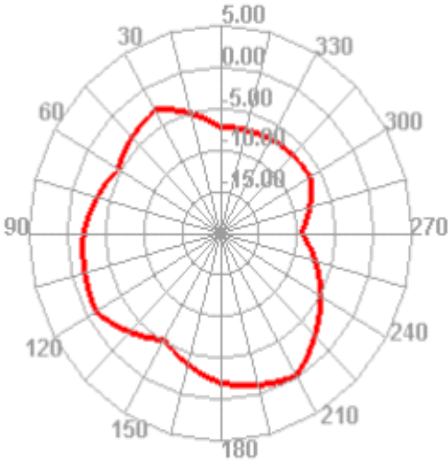
2500.000MHz E1
