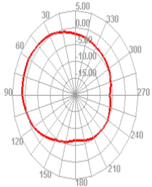
2450.000MHz H
