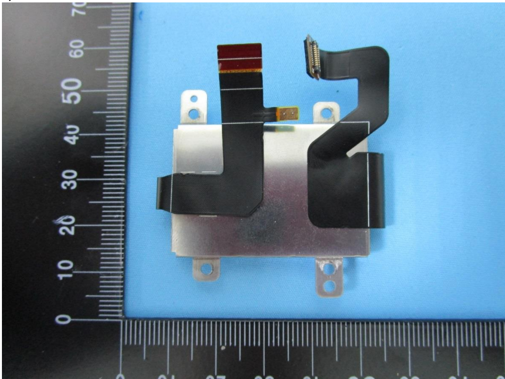
(24) EUT Photo
