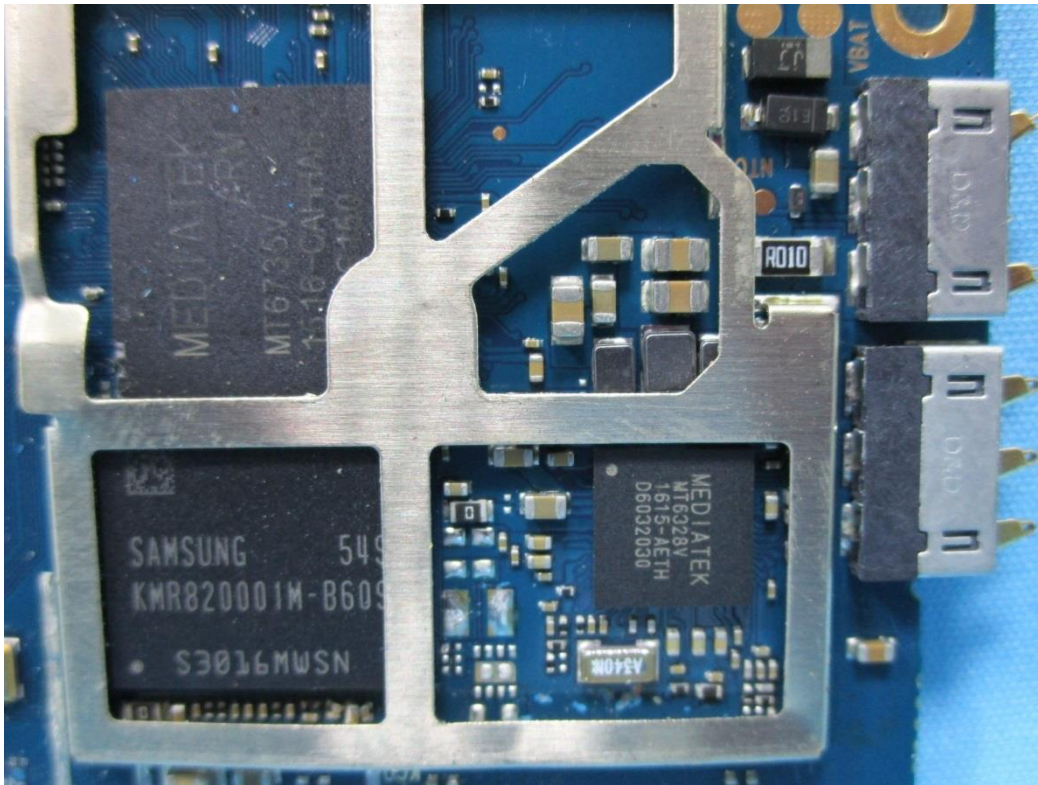
(12) EUT Photo
