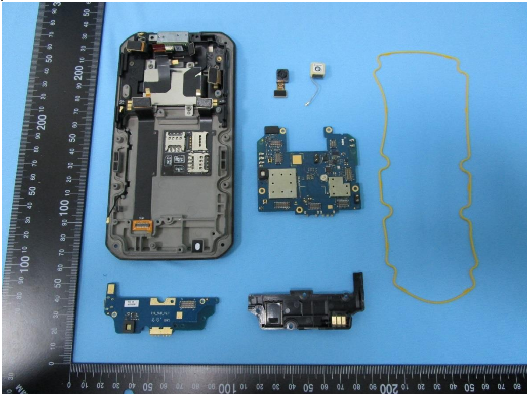
(2) EUT Photo
