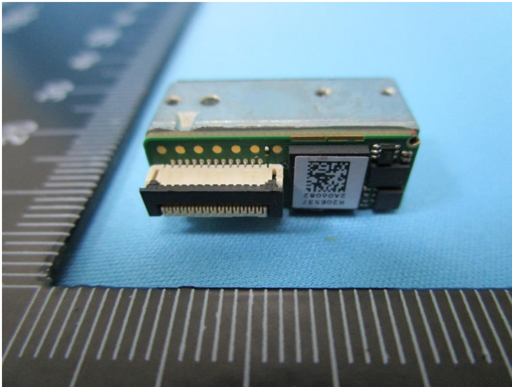
(30) EUT Photo
