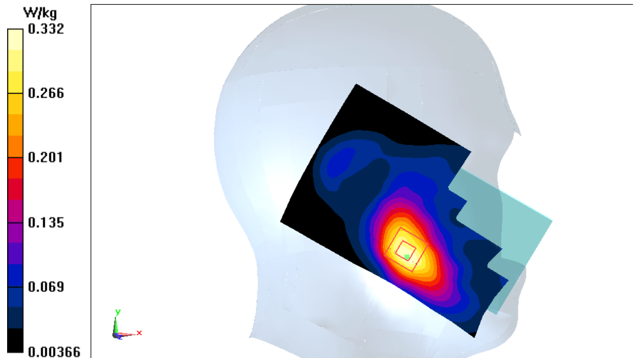
Fig.43 LTE Band66
