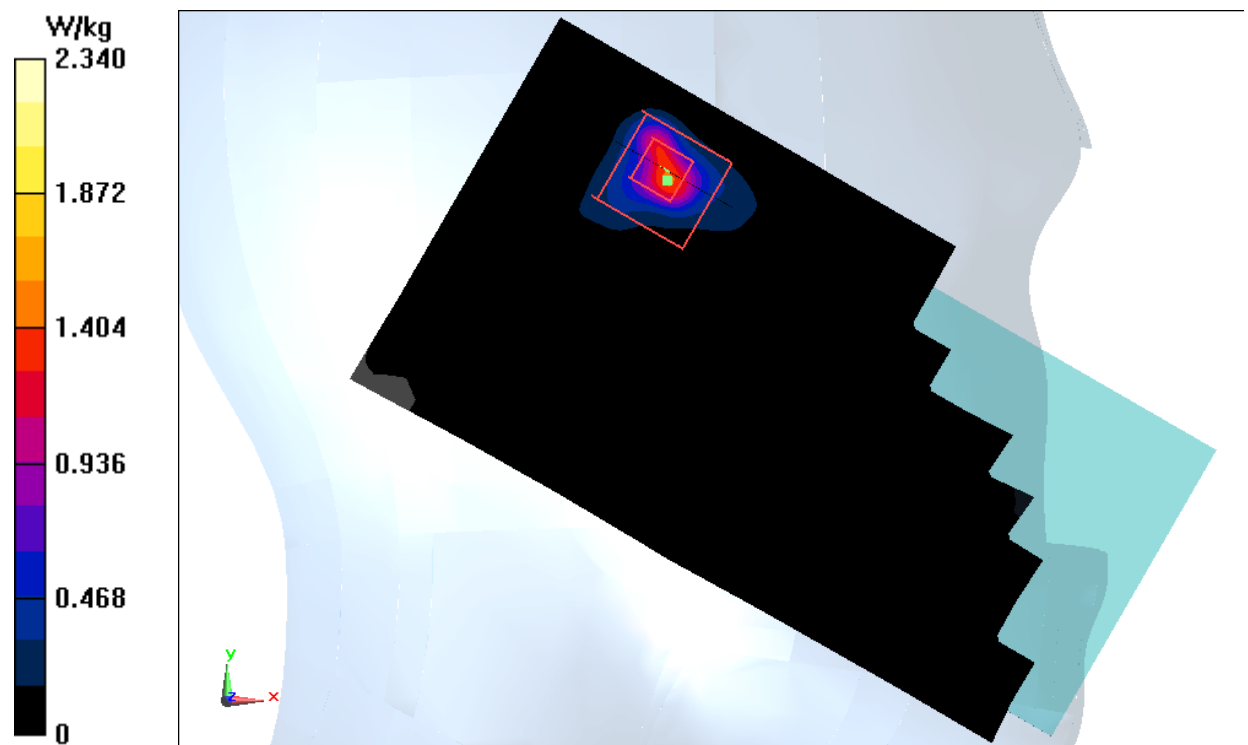
Fig.48 5GHz
