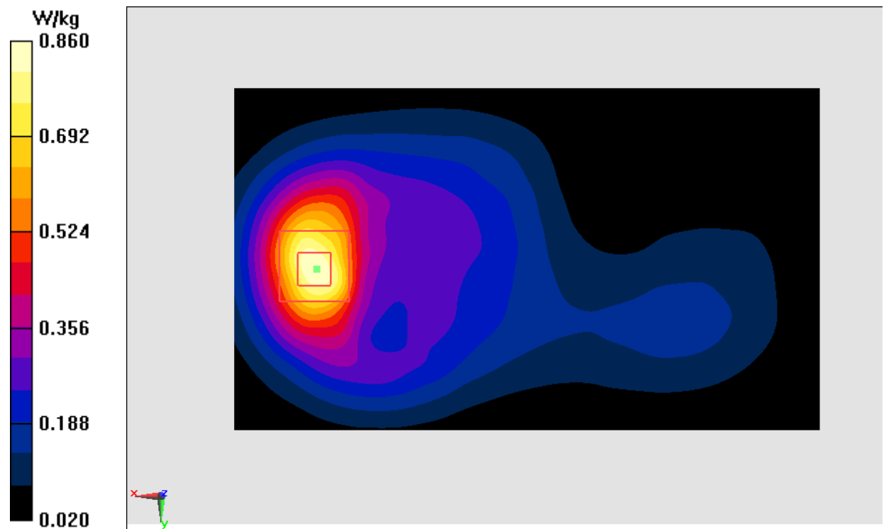
Fig.44 LTE Band66
