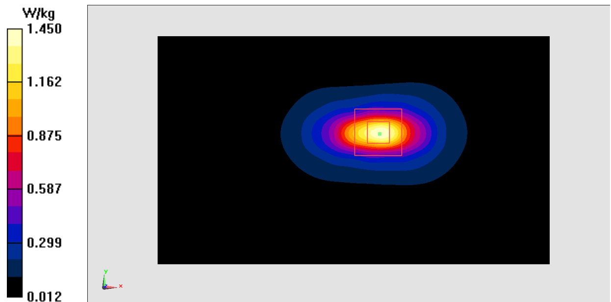
Fig.4 CDMA BC1
