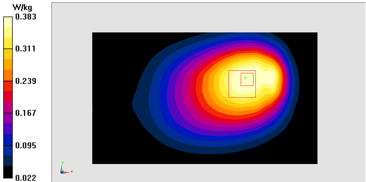
Fig.19 LTE Band17
