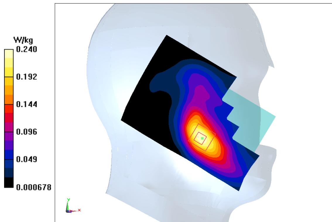
Fig.11 LTE Band4
