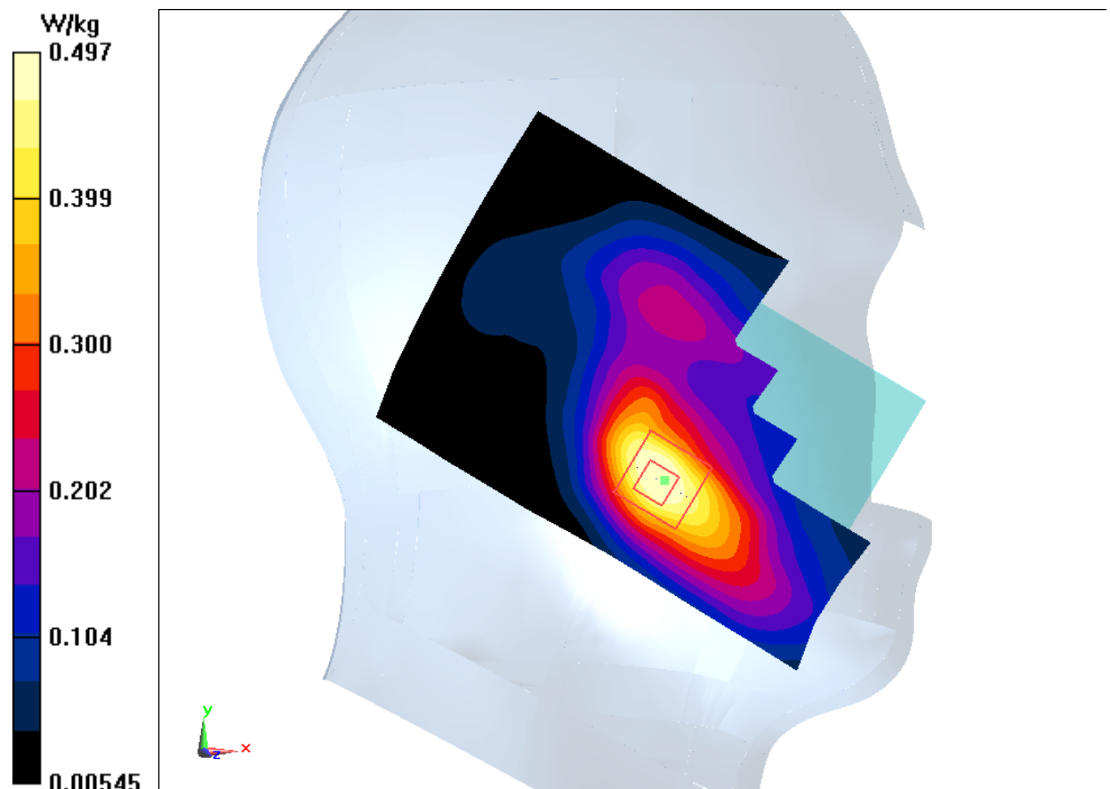
Fig.11 LTE Band2
