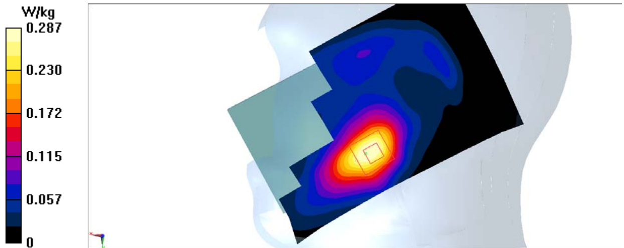
Fig.19 1700MHz
