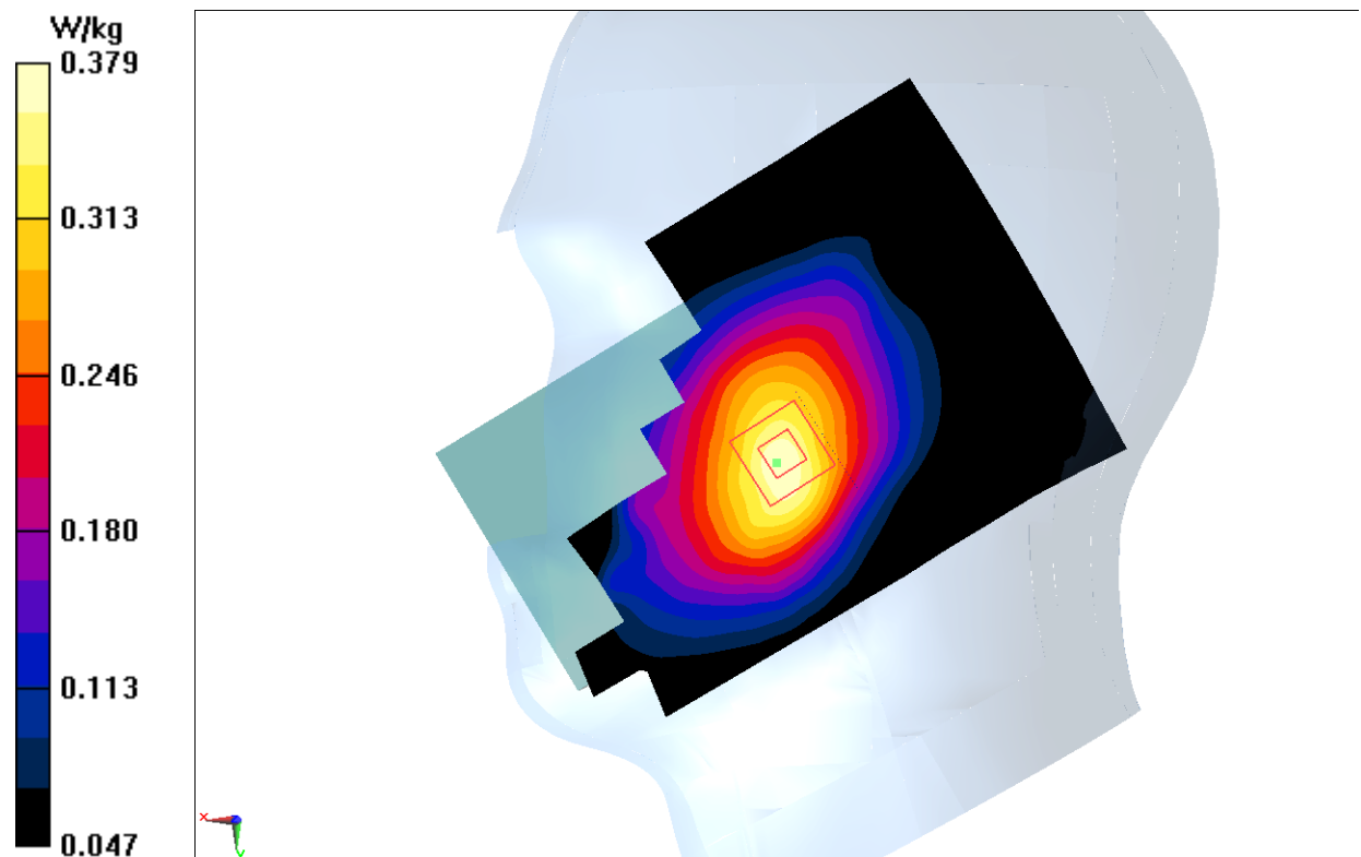
Fig.21 LTE Band5
