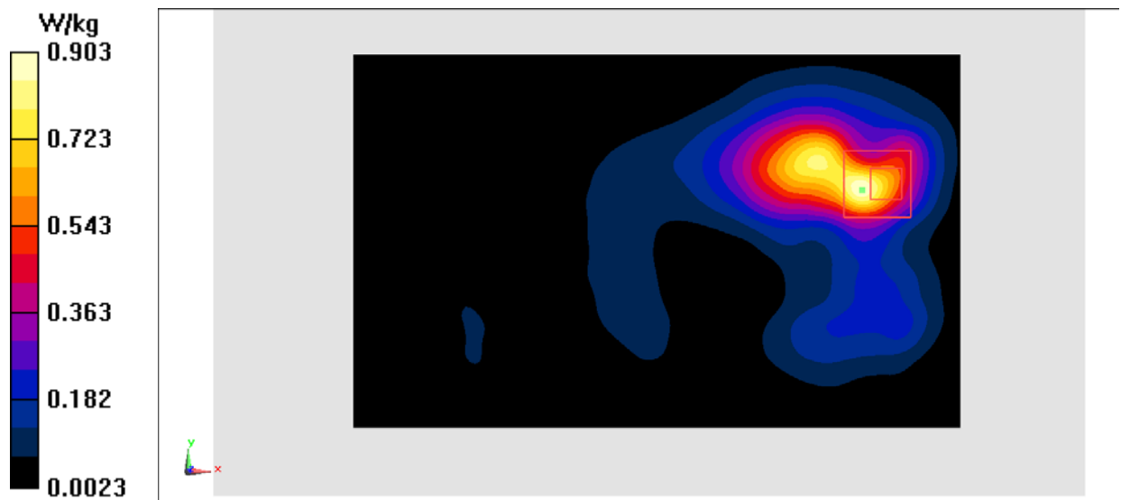
Fig.16 LTE Band7
