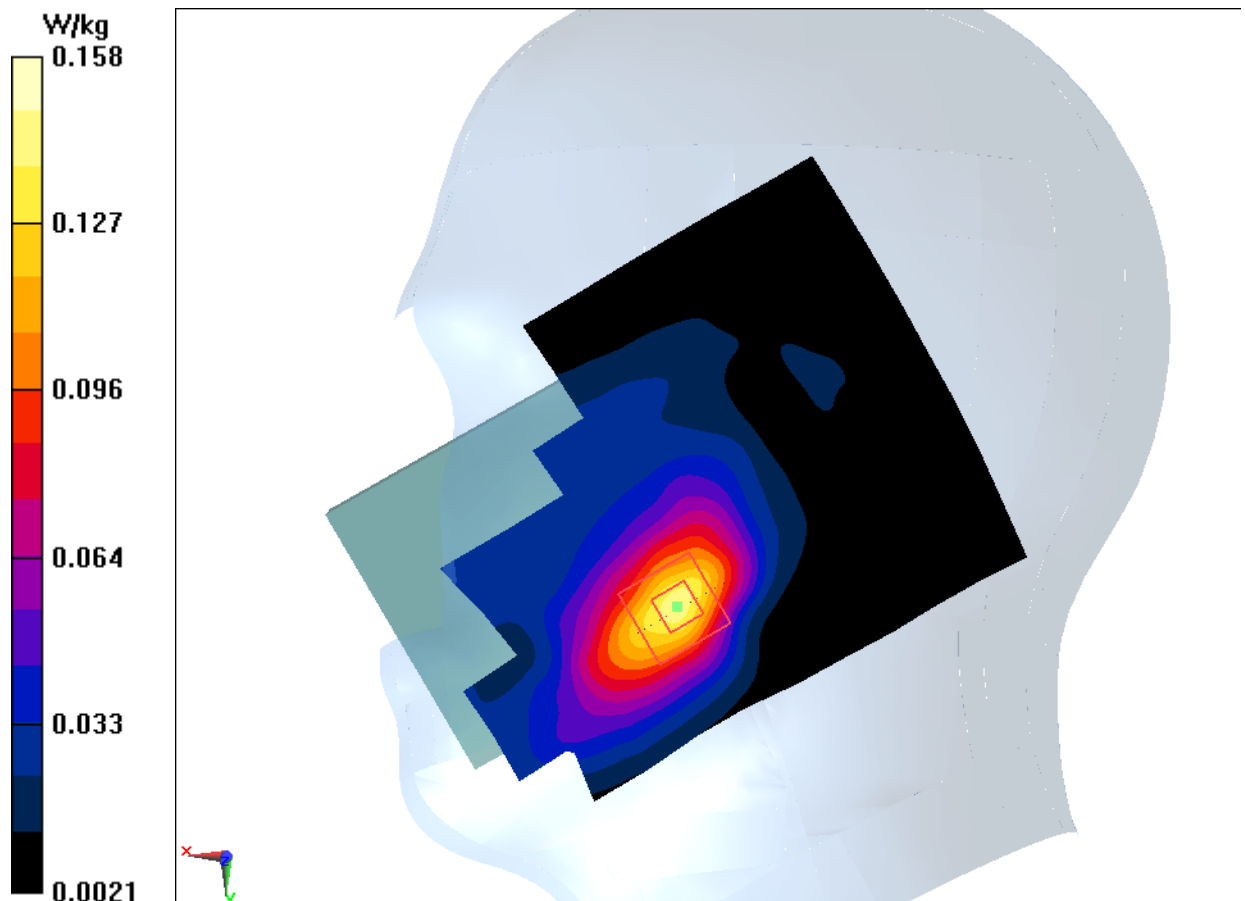
Fig.10 LTE Band2
