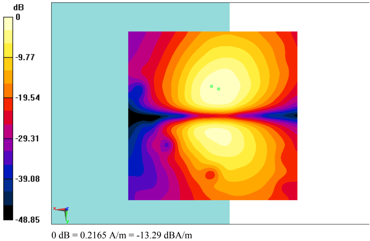
Fig B.9 T-Coil WCDMA 1900
