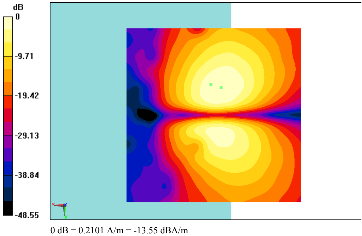
Fig B.5 T-Coil WCDMA 850
