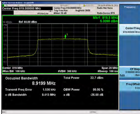
Band26-10MHz-QPSK-26740-50RB#0-8.9199
