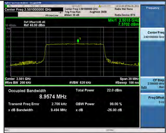
Band41-10MHz-QPSK-39700-50RB#0-8.9574
