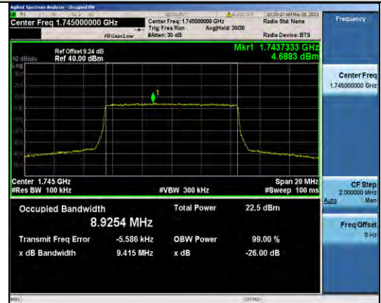
Band66-10MHz-QPSK-132322-50RB#0-8.9254
