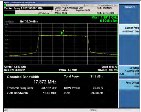
Band25-20MHz-QPSK-26365-100RB#0-17.872
