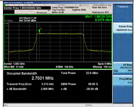
Band25-3MHz-QPSK-26365-15RB#0-2.7031
