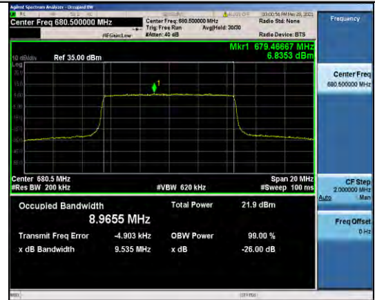
Band71-10MHz-QPSK-133297-50RB#0-8.9655
