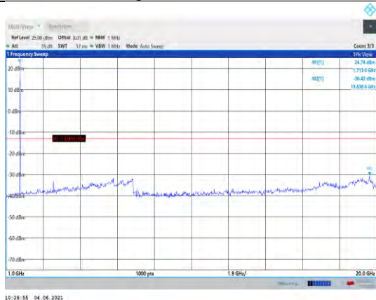
Band66-5MHz-QPSK-131997-1RB#0- Range2:1000~20000MHz
