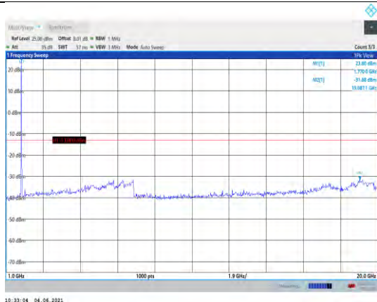
Band66-10MHz-QPSK-132622-1RB#0- Range2:1000~20000MHz
