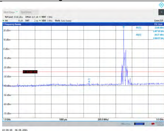
Band41-15MHz-QPSK-39725-1RB#0- Range2:1000~3000MHz
