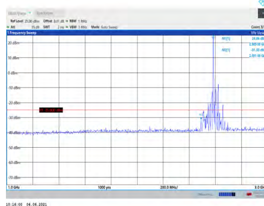
Band41-20MHz-QPSK-40620-1RB#0- Range2:1000~3000MHz
