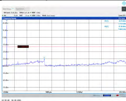
Band66-10MHz-QPSK-132022-1RB#0- Range2:1000~20000MHz
