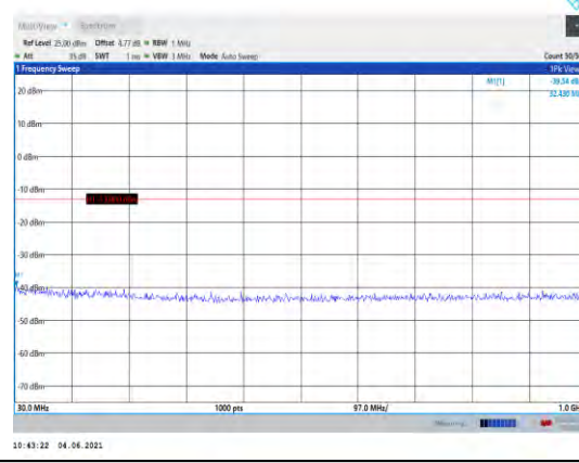
Band66-20MHz-QPSK-132572-1RB#0- Range1:30~1000MHz
