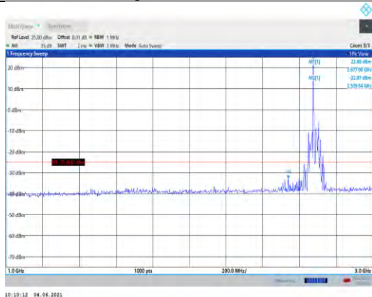
Band41-15MHz-QPSK-41515-1RB#0- Range2:1000~3000MHz
