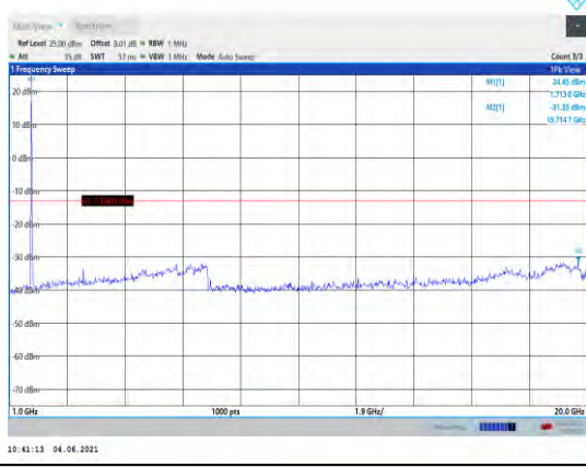
Band66-20MHz-QPSK-132072-1RB#0- Range2:1000~20000MHz
