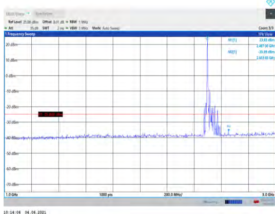
Band41-20MHz-QPSK-39750-1RB#0- Range2:1000~3000MHz
