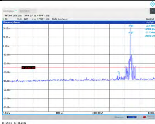
Band41-20MHz-QPSK-41490-1RB#0- Range2:1000~3000MHz
