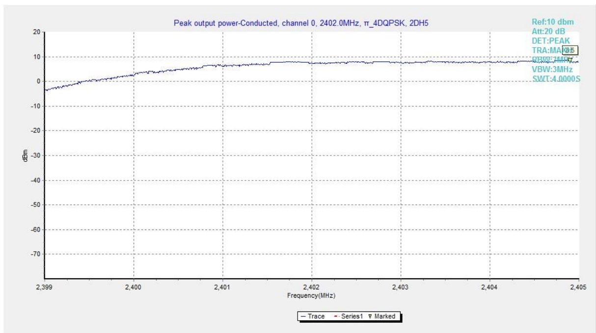
Fig. 4 RF output power ( \pi/4 DQPSK, Ch 0)
