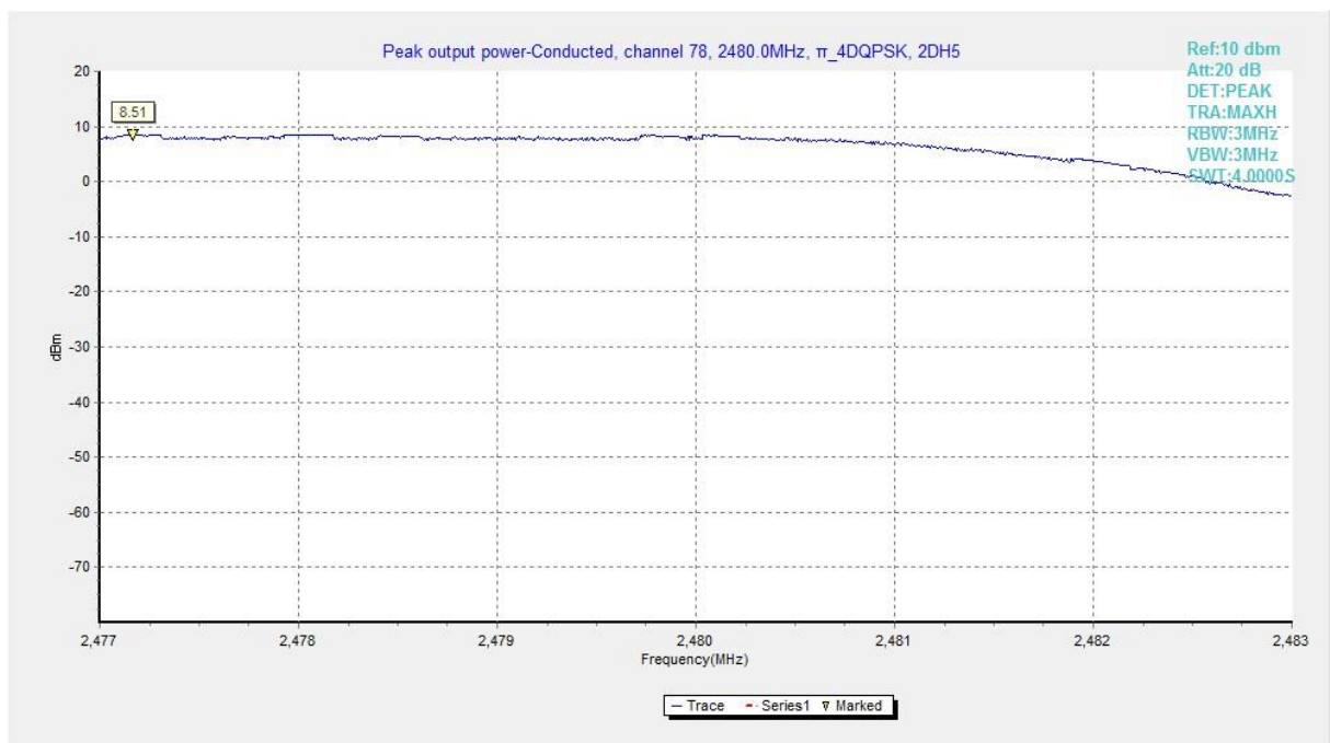
Fig. 6 RF output power ( \pi/4 DQPSK, Ch 78)
