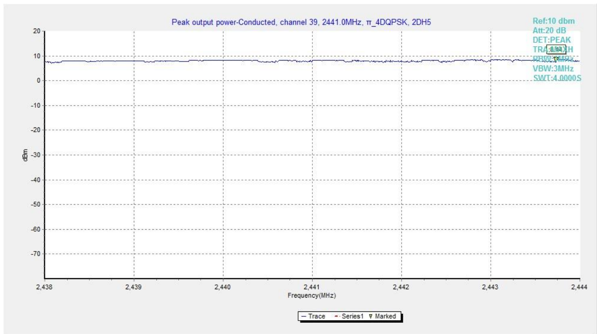
Fig. 5 RF output power ( \pi/4 DQPSK, Ch 39)
