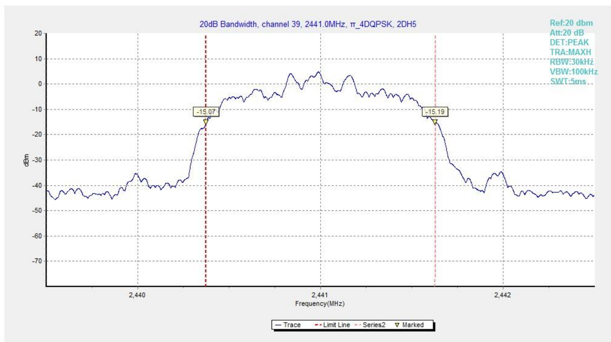
Fig. 65 20dB Bandwidth ( \pi /4 DQPSK, Ch 39)
