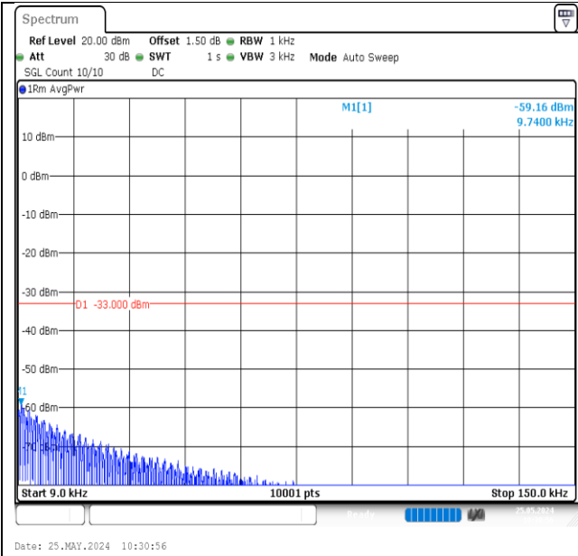
GSM850-128-5-0.009~0.15MHz-PASS
