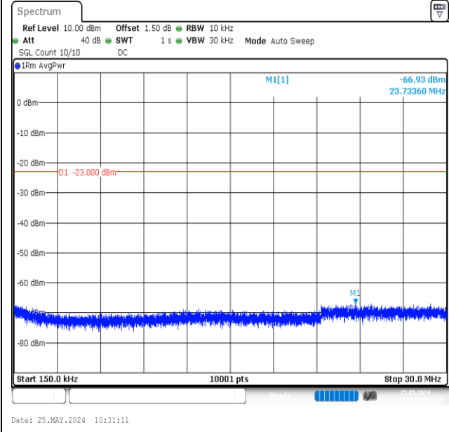
GSM850-128-5-0.15~30MHz-PASS
