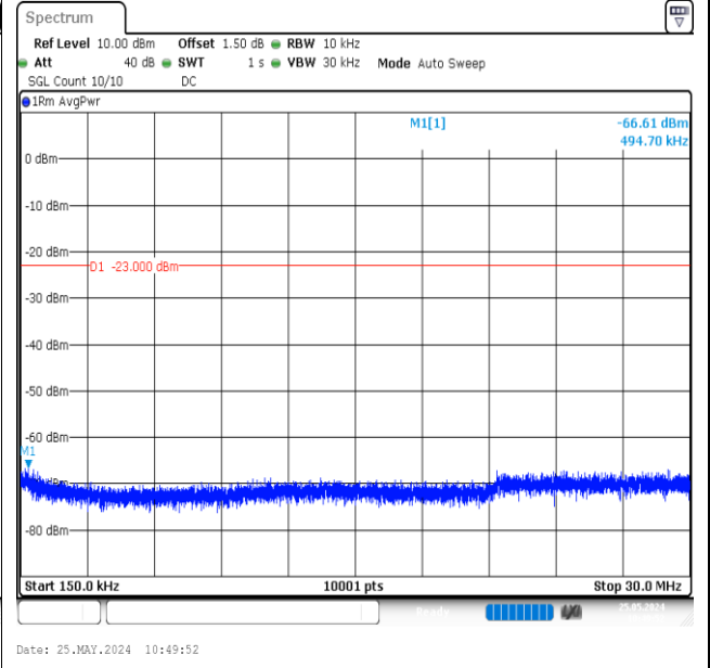
GPRS850-128-5-0.15~30MHz-PASS
