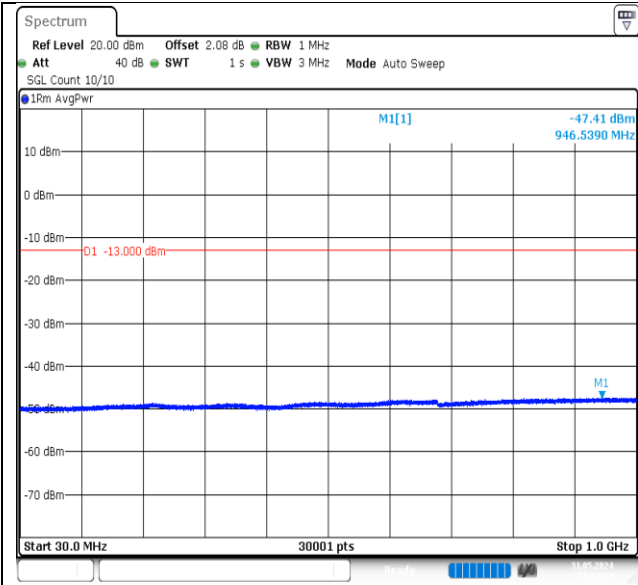
GPRS1900-810-0-30~1000MHz-PASS
