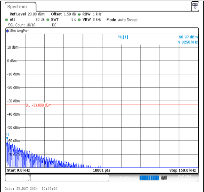
GPRS850-128-5-0.009~0.15MHz-PASS
