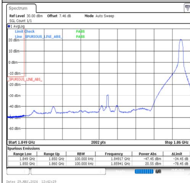
Band2-10MHz-QPSK-18650-1RB#49-PASS
