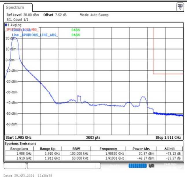
Band2-5MHz-QPSK-19175-1RB#0-PASS
