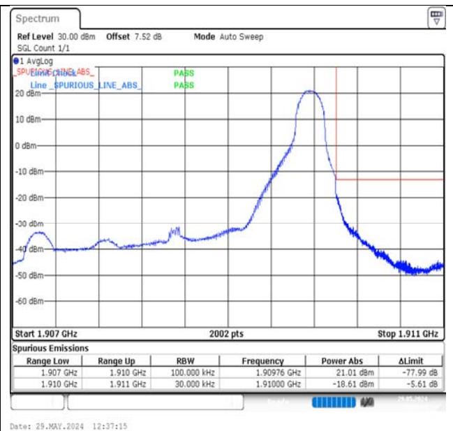
Band2-3MHz-QPSK-19185-1RB#14-PASS
