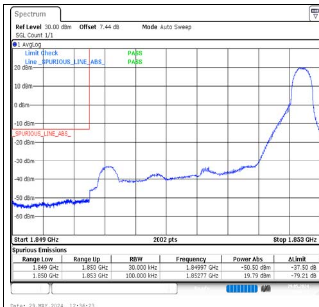
Band2-3MHz-16QAM-18615-1RB#14-PASS
