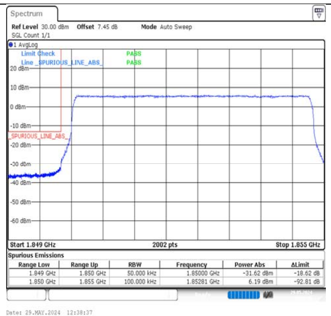
Band2-5MHz-QPSK-18625-25RB#0-PASS
