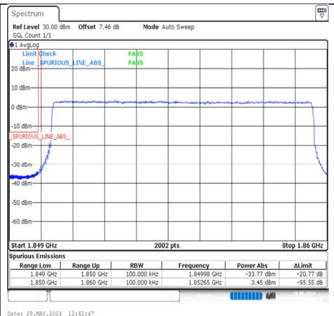
Band2-10MHz-QPSK-18650-50RB#0-PASS
