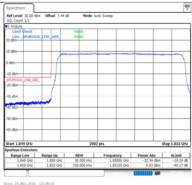
Band2-3MHz-QPSK-18615-15RB#0-PASS
