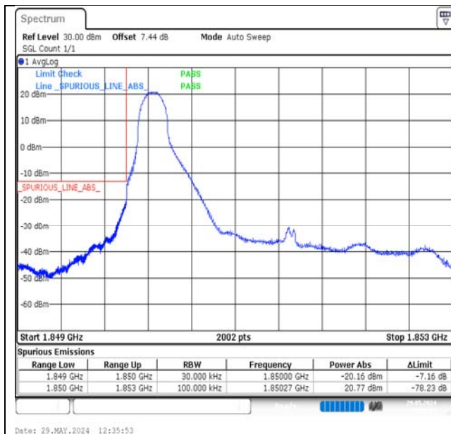
Band2-3MHz-QPSK-18615-1RB#0-PASS
