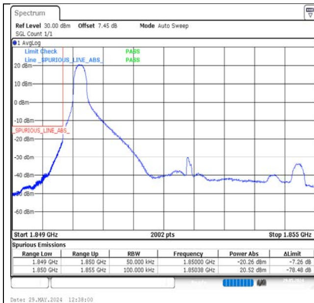
Band2-5MHz-QPSK-18625-1RB#0-PASS
