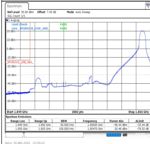
Band2-5MHz-QPSK-18625-1RB#24-PASS
