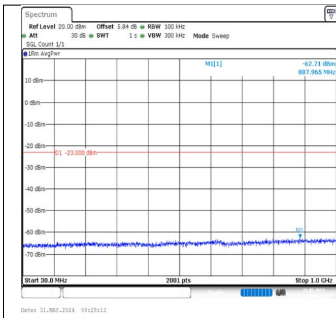
Band2-20MHz-QPSK-18700-1RB#0-30~1000-PASS
