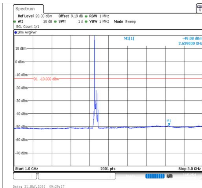
Band2-20MHz-QPSK-18700-1RB#0-1000~3000-PASS
