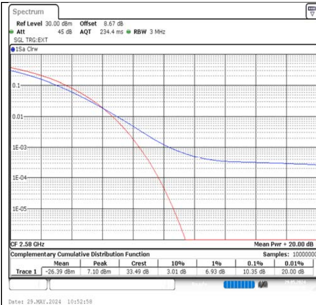
Band38-20MHz-QPSK-37850-1RB#0-PASS
