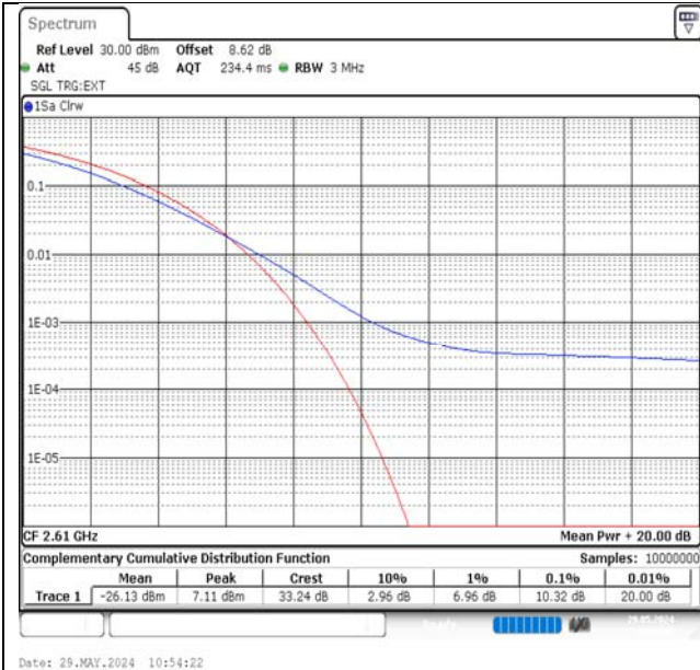
Band38-20MHz-QPSK-38150-1RB#0-PASS
