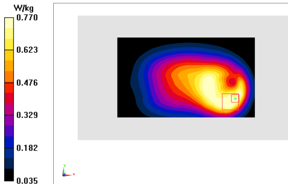
Fig.6 WCDMA 850
