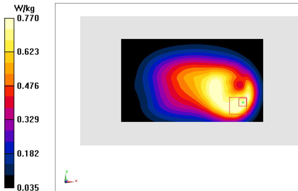
Fig.6 WCDMA 850
