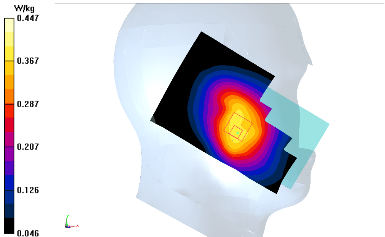
Fig.5 WCDMA 850
