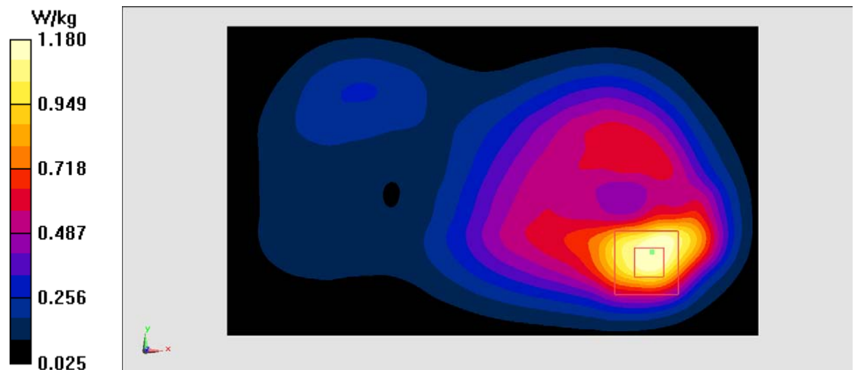
Fig.8 WCDMA1900
