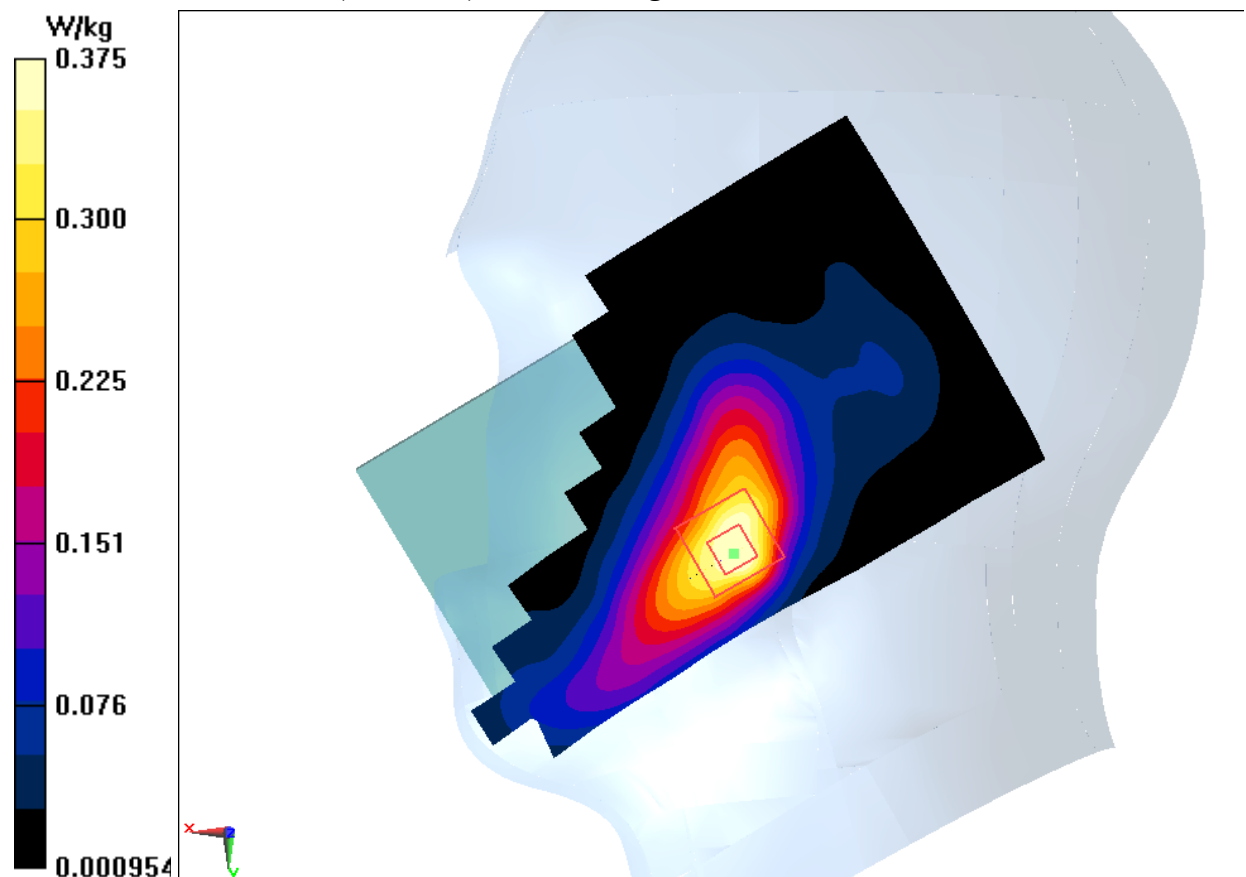
Fig.9 LTE Band7
