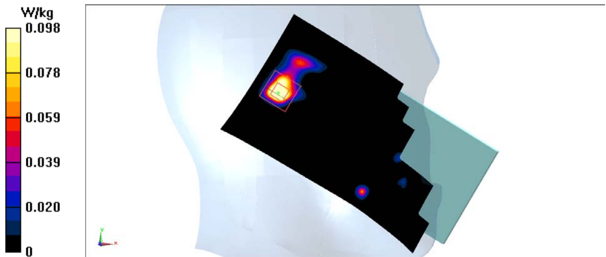
Fig.13 5GHz
