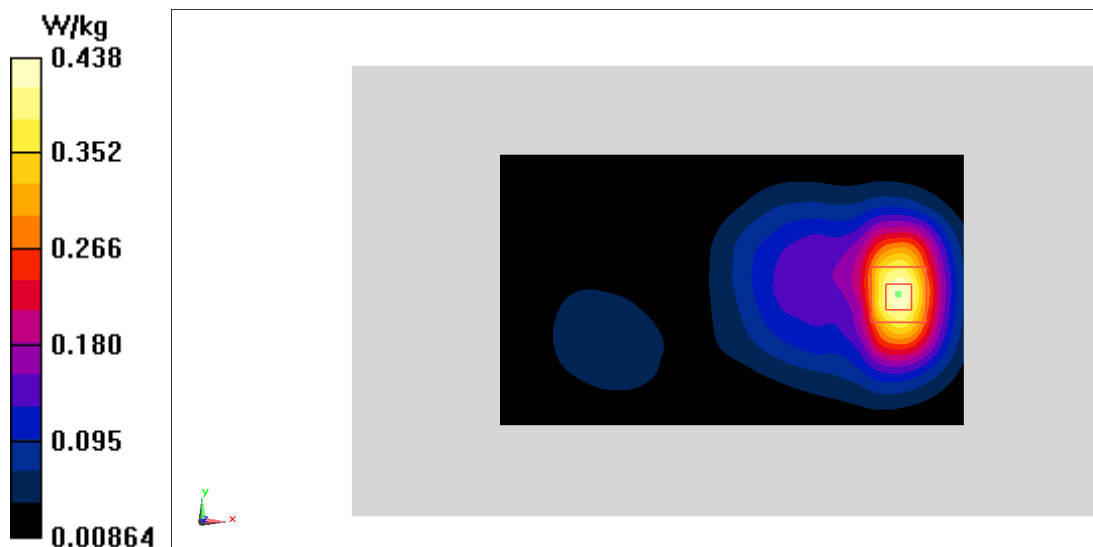
Fig.24 LTE Band66
