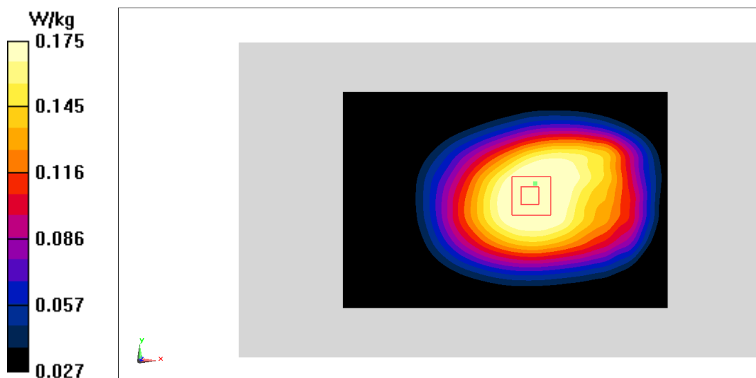
Fig.21 LTE Band13
