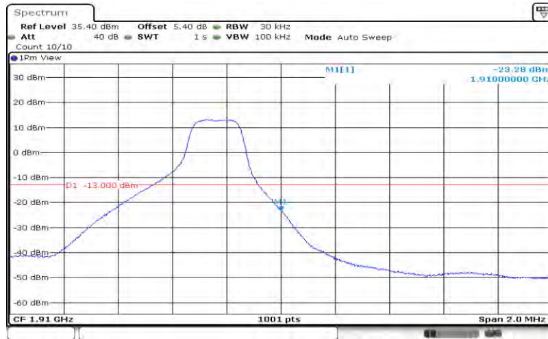
Band2-3MHz-QPSK-19185-15RB#0
