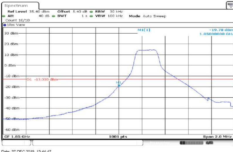
Band2-3MHz-16QAM-18615-15RB#0
