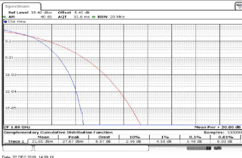
Band2-20MHz-16QAM-19100-100RB#0
