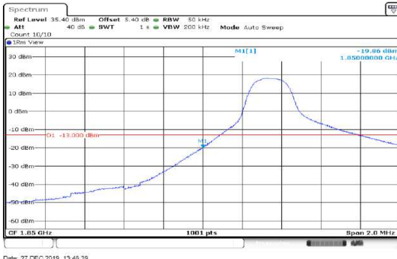
Band2-5MHz-QPSK-18625-25RB#0
