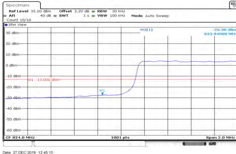
Band5-3MHz-QPSK-20635-1RB#14
