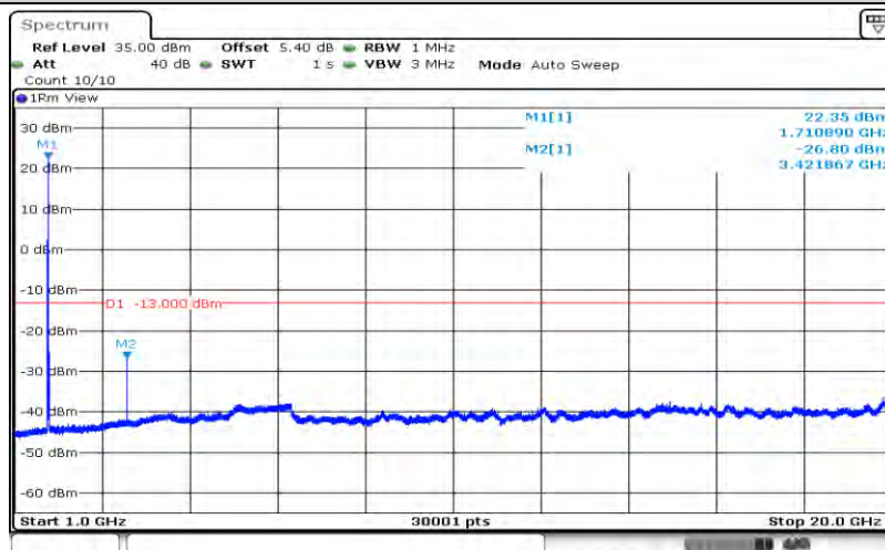
Band66-20MHz-QPSK-132072-1RB#0-Range2:1000~20000MHz
