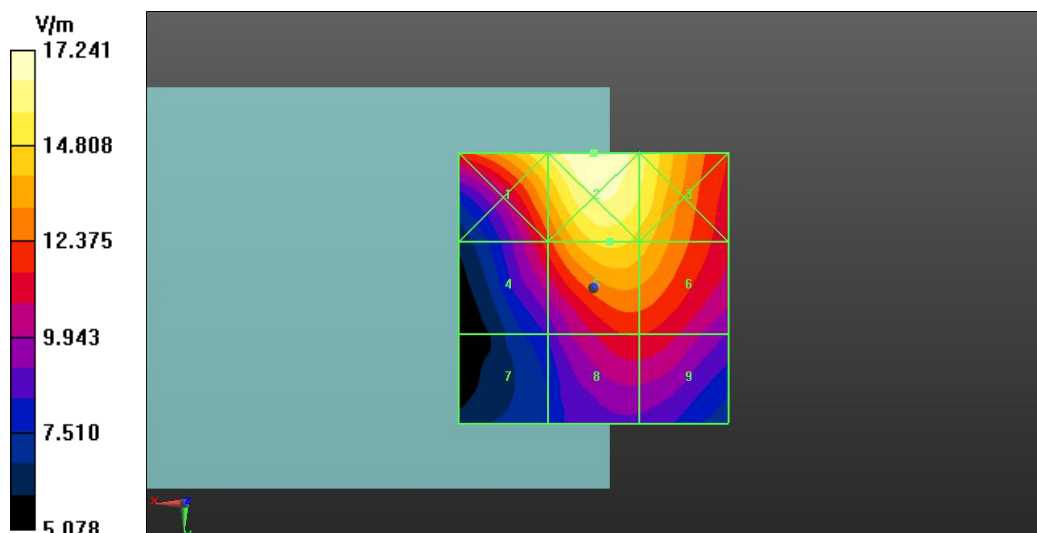
Fig A.4 HAC RF E-Field LTE-Band 41
