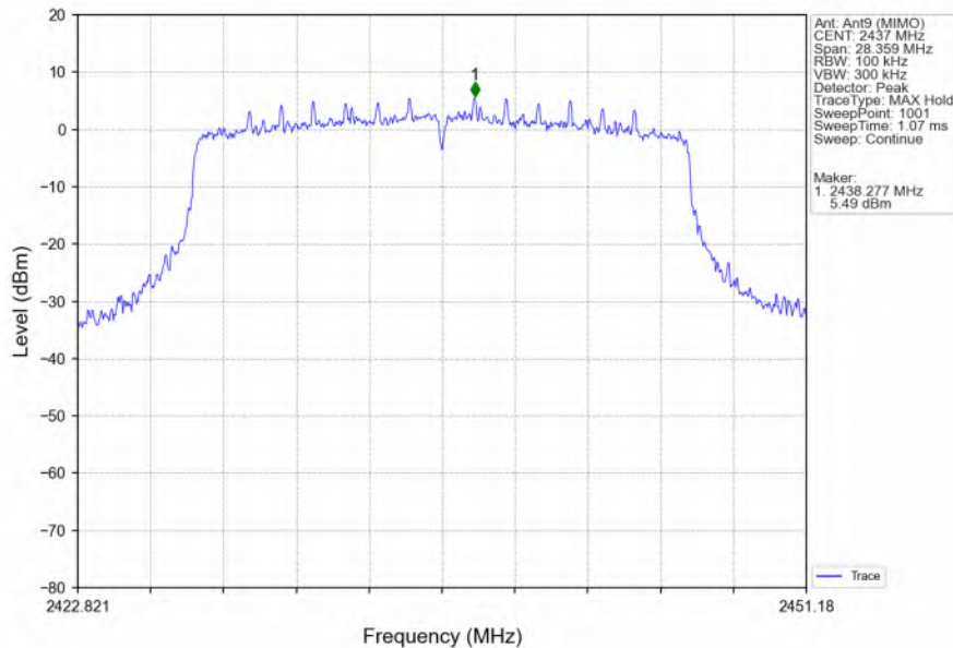
802.11ax(HEW20)_MCH_2437MHz_RU242_Left_Ant9 (MIMO)_NTNV
