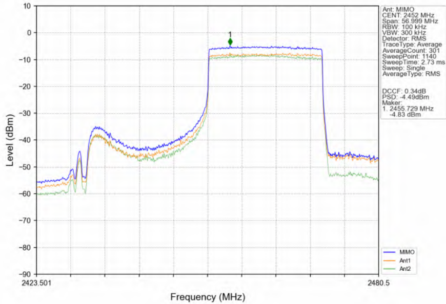
802.11ax(HEW40)_HCH_2452MHz_RU484_Left_Ant8 (MIMO)_NTNV
