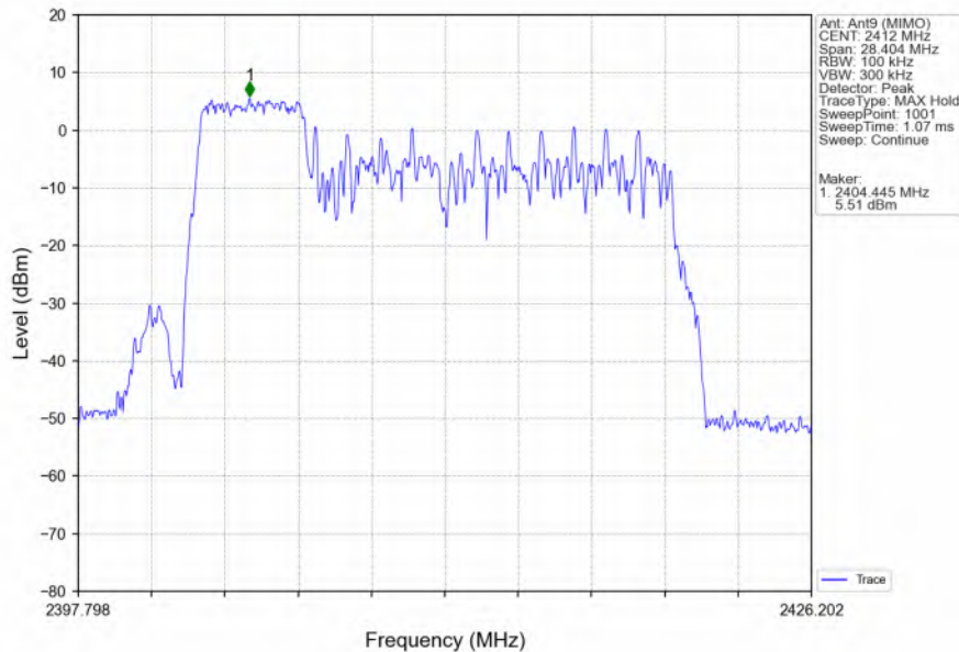
802.11ax(HEW20)_LCH_2412MHz_RU52_Left_Ant9 (MIMO)_NTNV
