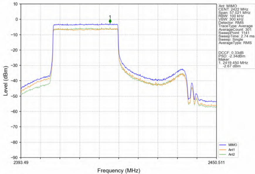
802.11ax(HEW40)_LCH_2422MHz_RU484_Left_Ant8 (MIMO)_NTNV
