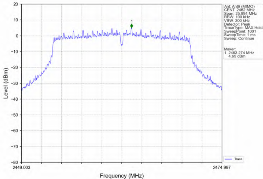
802.11n(HT20)_HCH_2462MHz_Ant9 (MIMO)_NTNV
