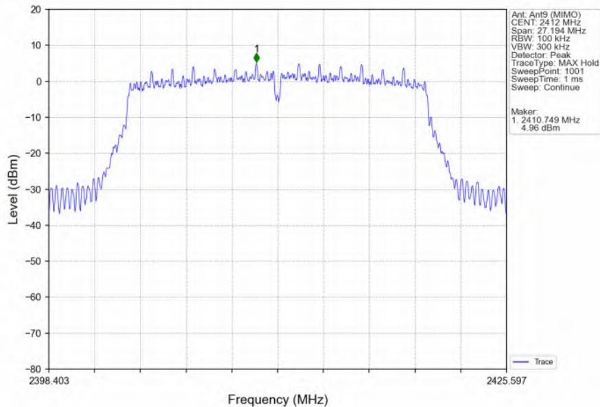
802.11n(HT20)_LCH_2412MHz_Ant9 (MIMO)_NTNV
