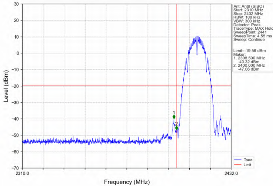
802.11b_LCH_2412MHz_Ant8 (SISO)_NTNV
