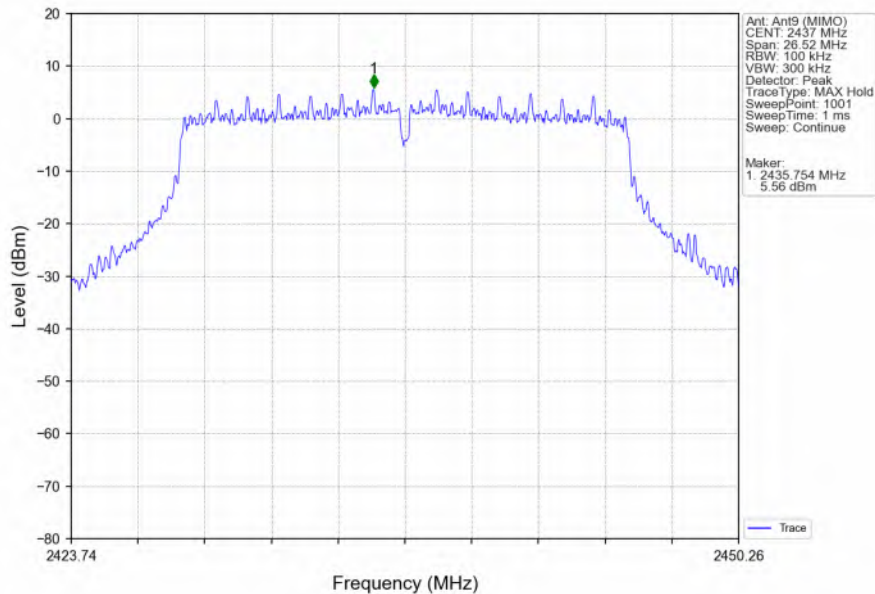
802.11n(HT20)_MCH_2437MHz_Ant9 (MIMO)_NTNV
