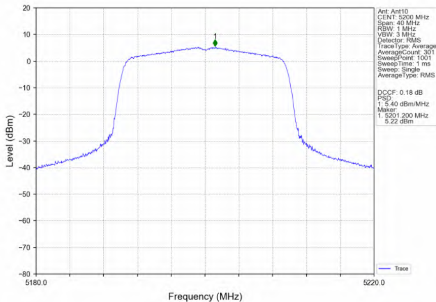
802.11ax(HEW20)_MCH_5200MHz_RU242_Left_Ant10_NTNV
