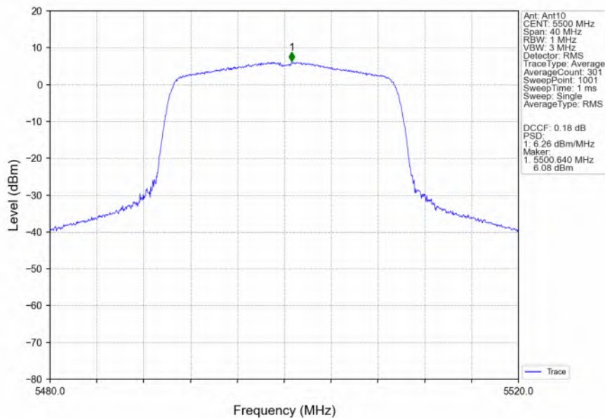
802.11ax(HEW20)_LCH_5500MHz_RU242_Left_Ant10_NTNV
