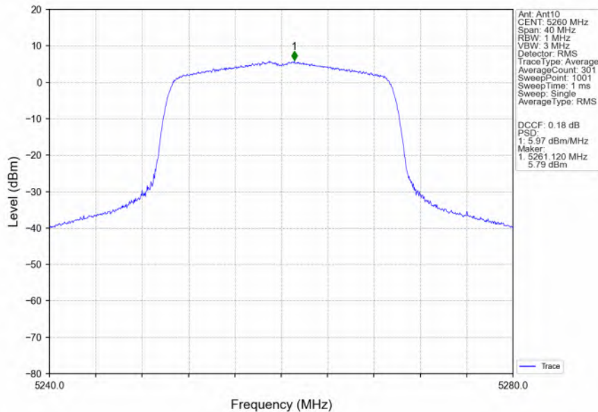
802.11ax(HEW20)_LCH_5260MHz_RU242_Left_Ant10_NTNV
