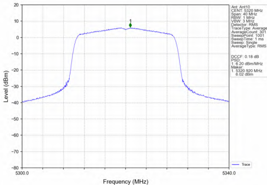
802.11ax(HEW20)_HCH_5320MHz_RU242_Left_Ant10_NTNV
