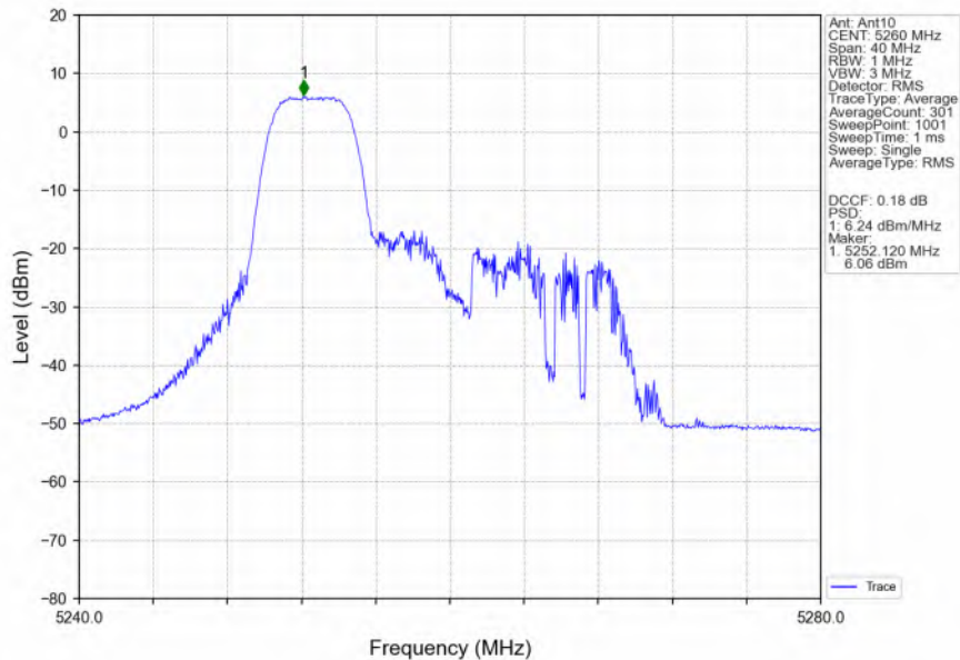
802.11ax(HEW20)_LCH_5260MHz_RU52_Left_Ant10_NTNV
