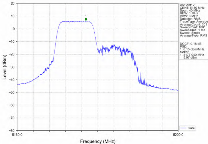
802.11ax(HEW20)_LCH_5180MHz_RU106_Left_Ant12_NTNV
