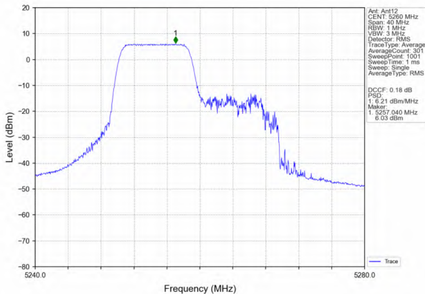
802.11ax(HEW20)_LCH_5260MHz_RU106_Left_Ant12_NTNV
