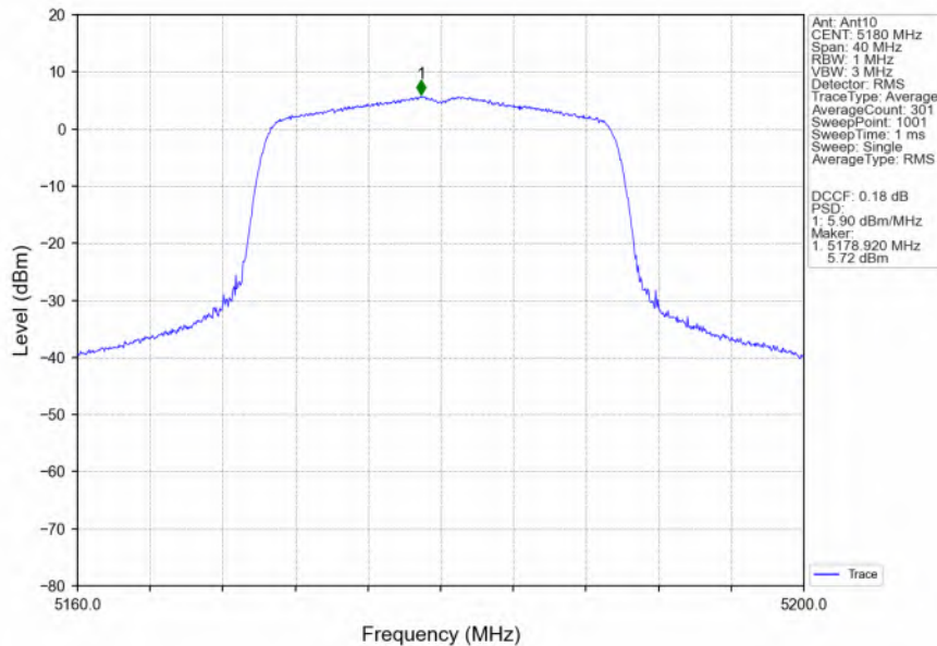
802.11ax(HEW20)_LCH_5180MHz_RU242_Left_Ant10_NTNV
