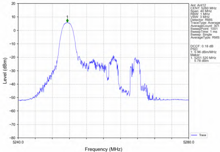
802.11ax(HEW20)_LCH_5260MHz_RU26_Left_Ant12_NTNV
