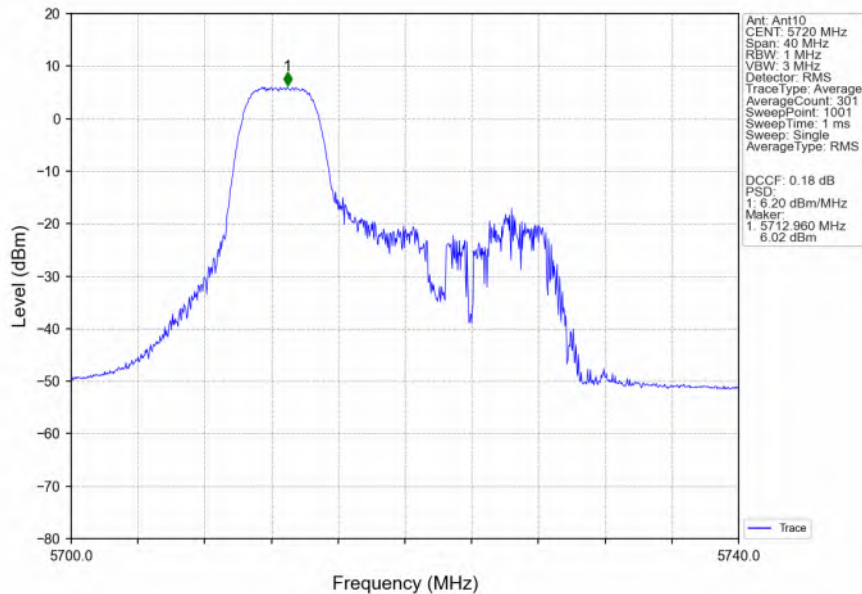
802.11ax(HEW20)_HCH_5720MHz_RU52_Left_Ant10_NTNV
