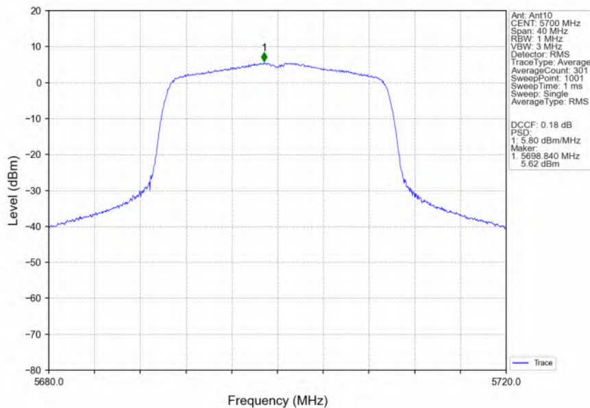
802.11ax(HEW20)_HCH_5700MHz_RU242_Left_Ant10_NTNV
