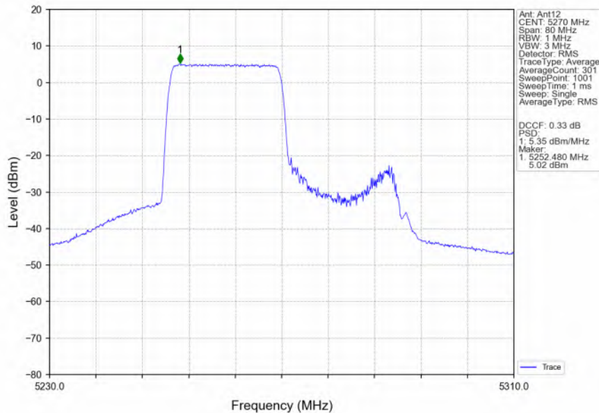
802.11ax(HEW40)_LCH_5270MHz_RU242_Left_Ant12_NTNV
