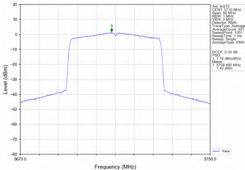
802.11ax(HEW40)_HCH_5710MHz_RU484_Left_Ant10_NTNV
