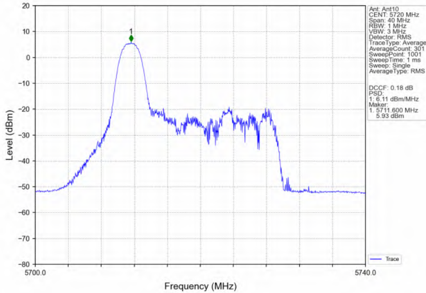
802.11ax(HEW20)_HCH_5720MHz_RU26_Left_MIMO_NTNV
