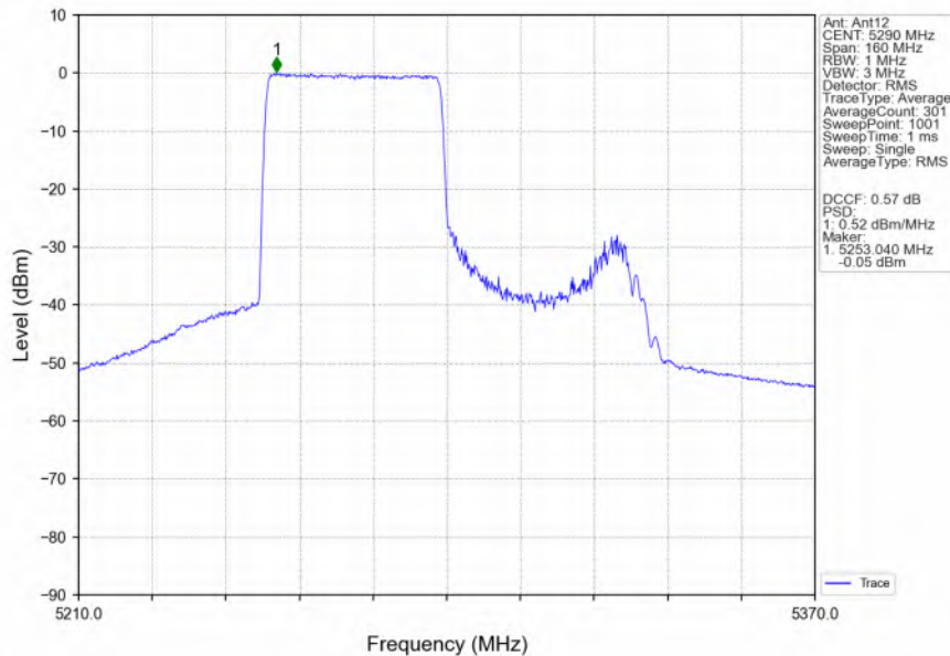
802.11ax(HEW80)_MCH_5290MHz_RU484_Left_Ant12_NTNV
