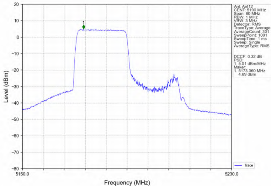
802.11ax(HEW40)_LCH_5190MHz_RU242_Left_Ant12_NTNV
