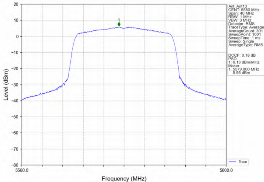
802.11ax(HEW20)_MCH_5580MHz_RU242_Left_Ant10_NTNV
