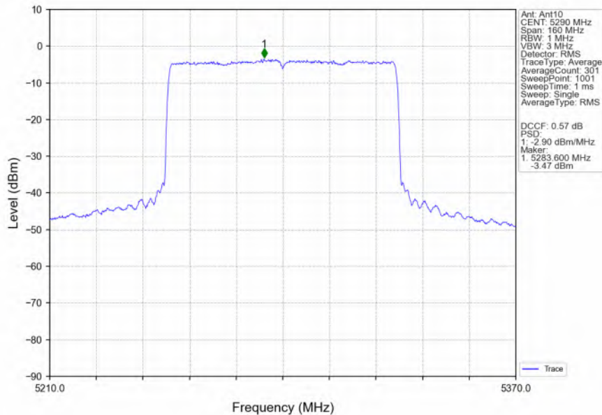
802.11ax(HEW80)_MCH_5290MHz_RU996_Left_Ant10_NTNV
