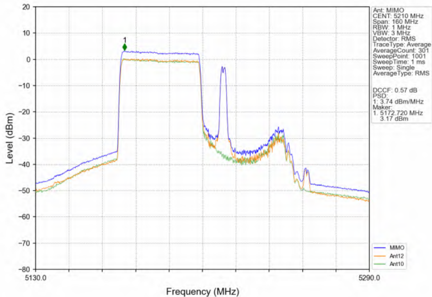
802.11ax(HEW80)_MCH_5210MHz_RU484_Left_MIMO_NTNV
