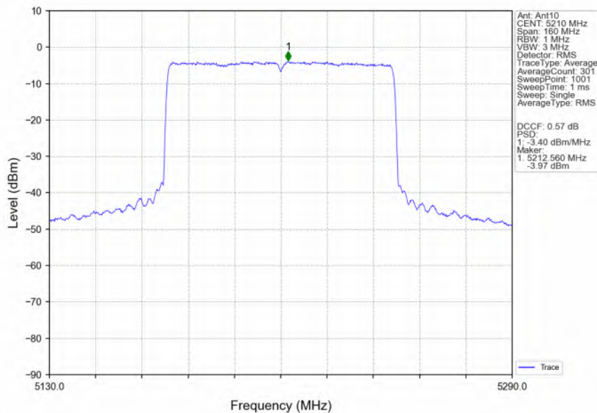
802.11ax(HEW80)_MCH_5210MHz_RU996_Left_Ant10_NTNV
