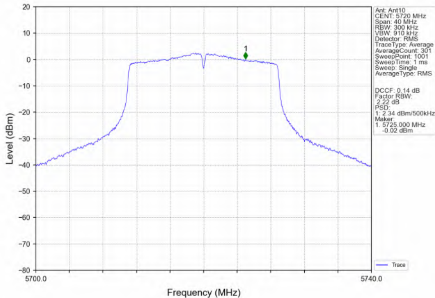
802.11ac(VHT20)_HCH_5720MHz_Ant10_NTNV
