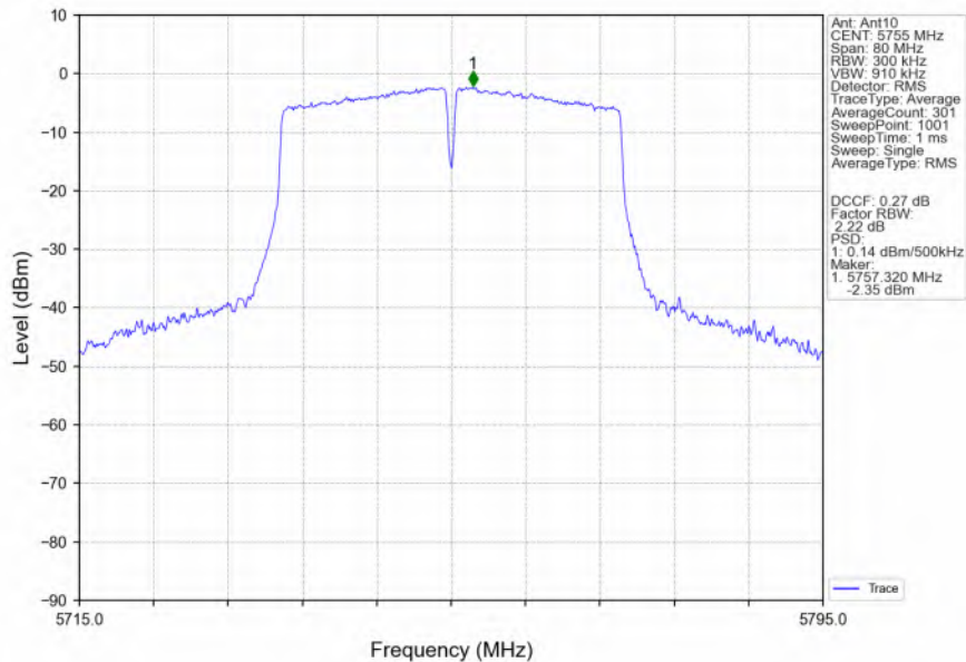
802.11n(HT40)_LCH_5755MHz_Ant10_NTNV
