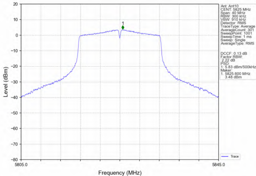
802.11a_HCH_5825MHz_Ant10_NTNV
