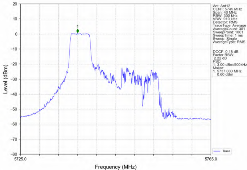
802.11ax(HEW20)_LCH_5745MHz_RU52_Left_Ant12_NTNV
