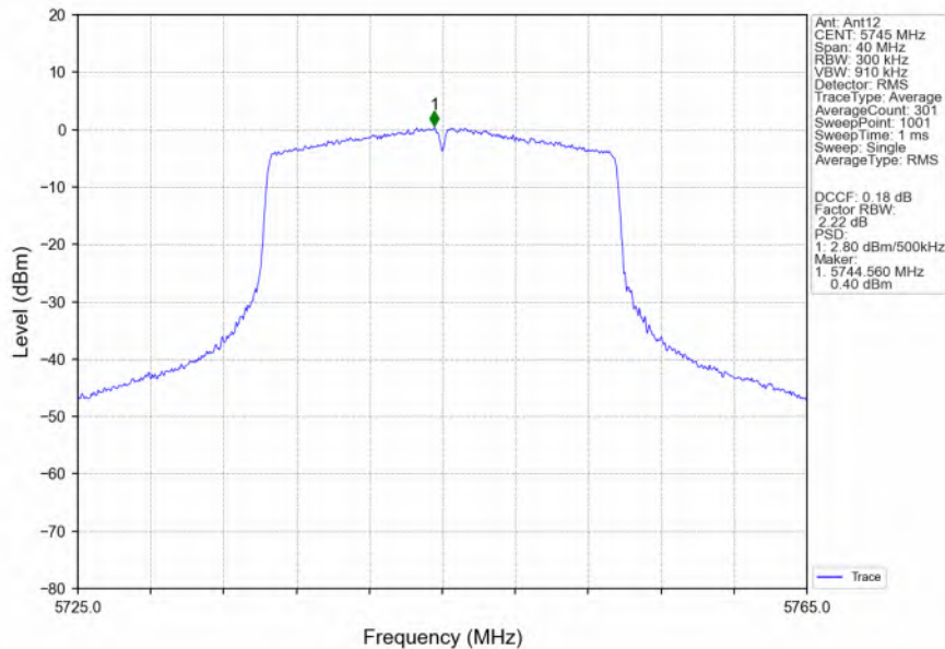
802.11ax(HEW20)_LCH_5745MHz_RU242_Left_Ant12_NTNV
