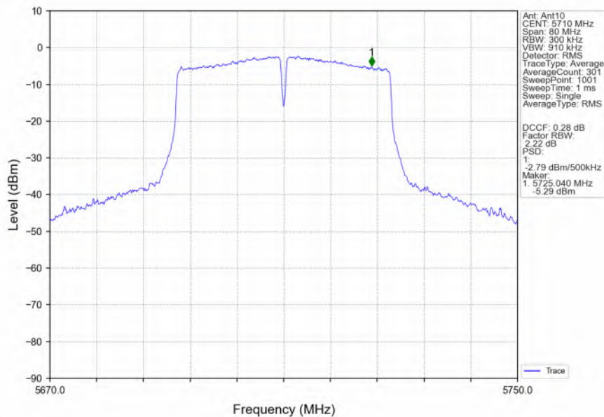
802.11n(HT40)_HCH_5710MHz_Ant10_NTNV
