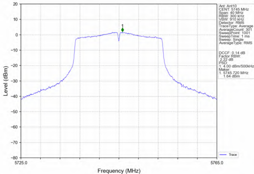
802.11n(HT20)_LCH_5745MHz_Ant10_NTNV
