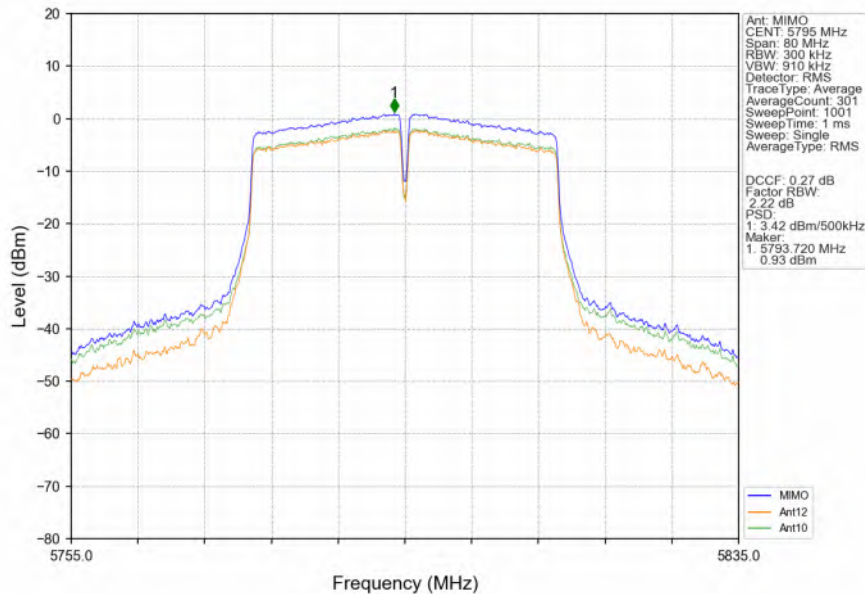
802.11n(HT40)_HCH_5795MHz_MIMO_NTNV
