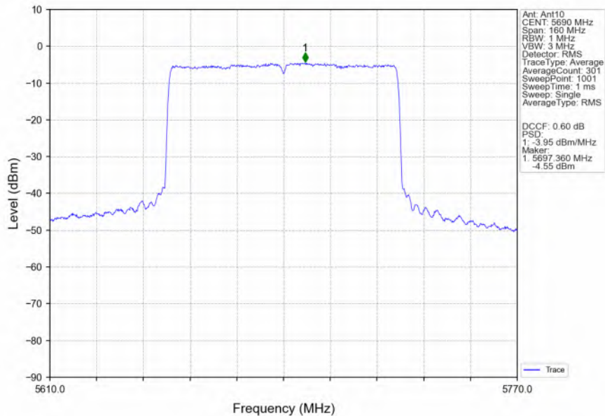
802.11ax(HEW80)_HCH_5690MHz_RU996_Left_Ant10_NTNV
