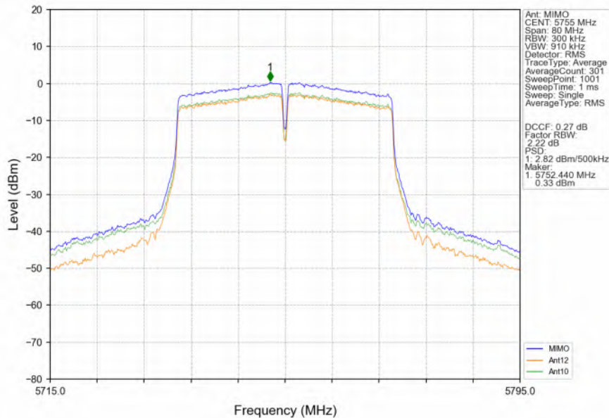
802.11ac(VHT40)_LCH_5755MHz_MIMO_NTNV
