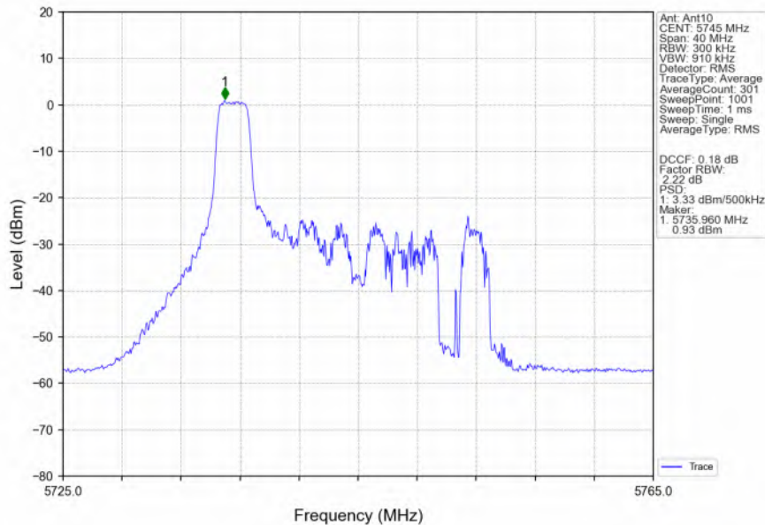
802.11ax(HEW20)_LCH_5745MHz_RU26_Left_Ant10_NTNV
