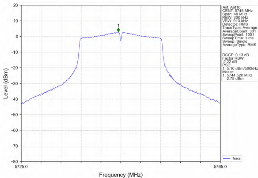
802.11a_LCH_5745MHz_Ant10_NTNV
