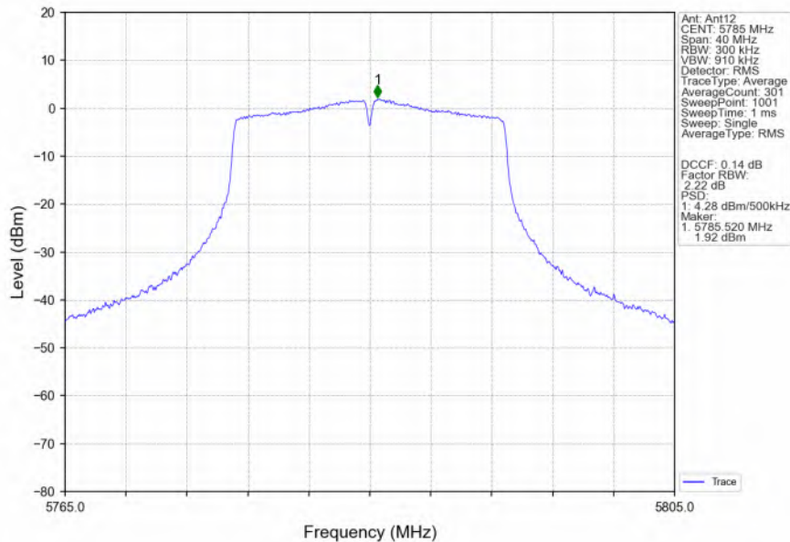
802.11n(HT20)_MCH_5785MHz_Ant12_NTNV
