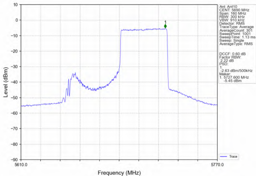
802.11ax(HEW80)_HCH_5690MHz_RU484_Right_Ant10_NTNV
