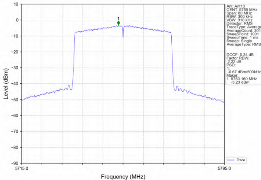
802.11ax(HEW40)_LCH_5755MHz_RU484_Left_Ant10_NTNV
