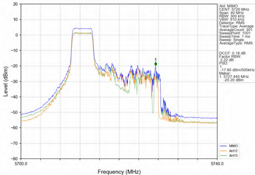
802.11ax(HEW20)_HCH_5720MHz_RU52_Left_MIMO_NTNV
