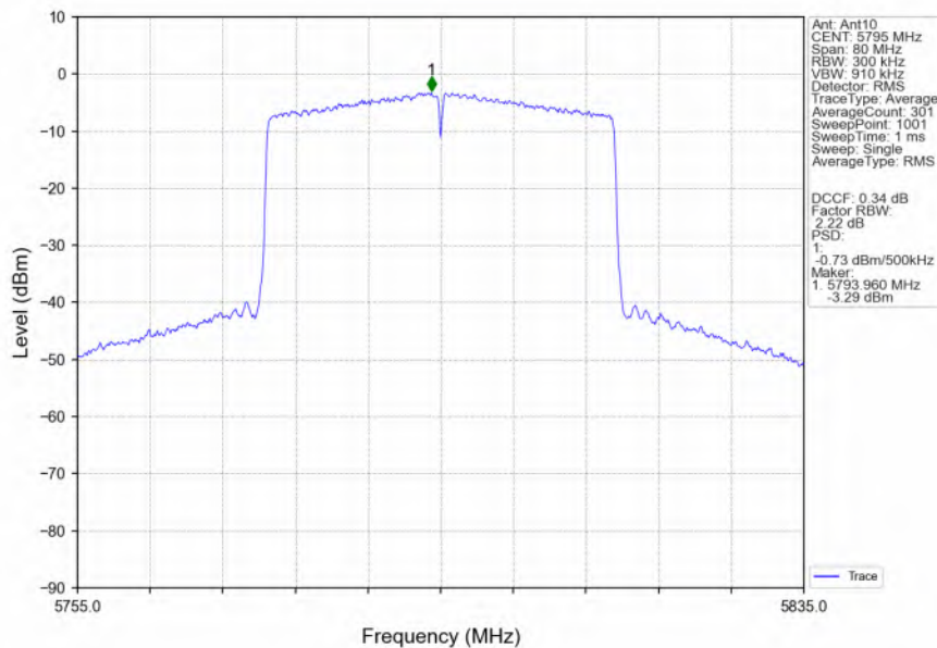
802.11ax(HEW40)_HCH_5795MHz_RU484_Left_Ant10_NTNV
