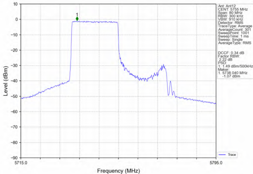
802.11ax(HEW40)_LCH_5755MHz_RU242_Left_Ant12_NTNV
