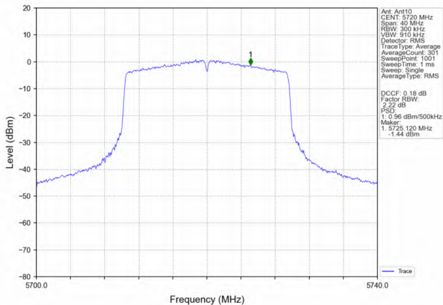
802.11ax(HEW20)_HCH_5720MHz_RU242_Left_Ant10_NTNV
