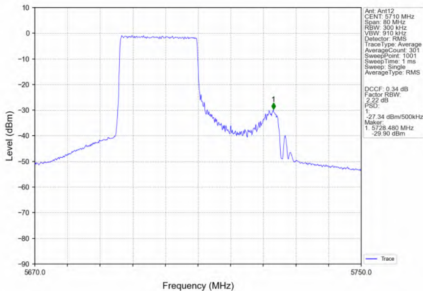
802.11ax(HEW40)_HCH_5710MHz_RU242_Left_Ant12_NTNV
