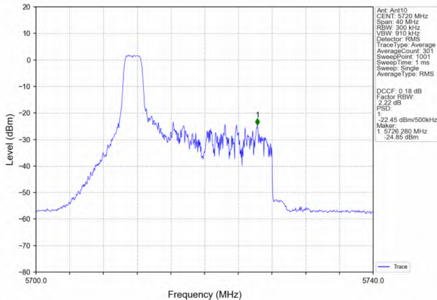
802.11ax(HEW20)_HCH_5720MHz_RU26_Left_Ant10_NTNV
