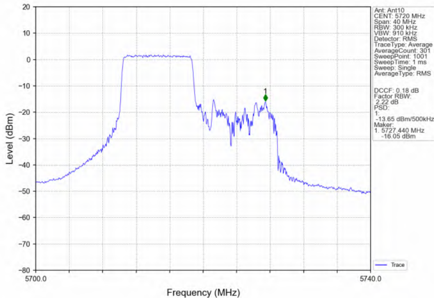
802.11ax(HEW20)_HCH_5720MHz_RU106_Left_Ant10_NTNV
