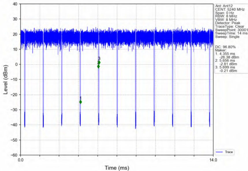
802.11n(HT20)_HCH_5240MHz_Ant12_NTNV
