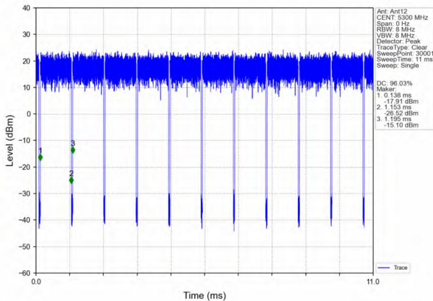
802.11ax(HEW20)_MCH_5300MHz_RU242_Left_Ant12_NTNV
