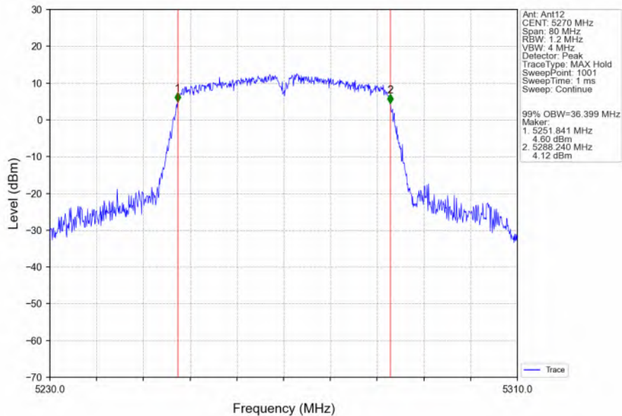
802.11ac(VHT40)_LCH_5270MHz_Ant12_NTNV
