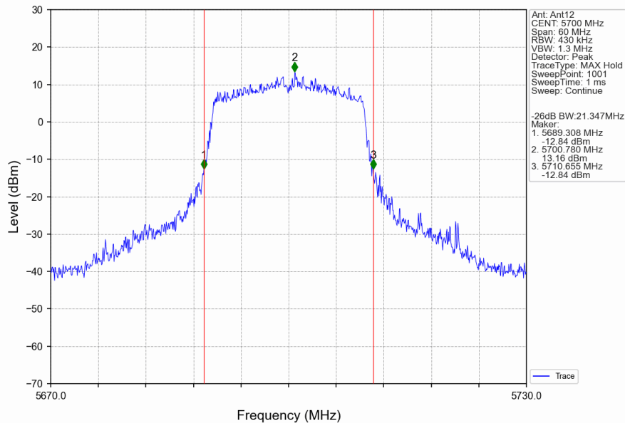
802.11ax(HEW20)_HCH_5700MHz_RU242_Left_Ant12_NTNV
