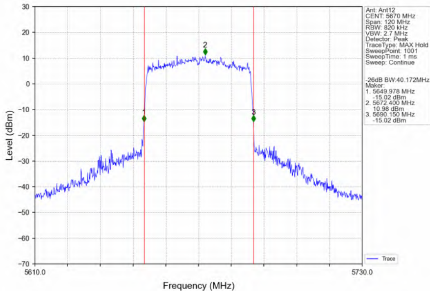
802.11ax(HEW40)_HCH_5670MHz_RU484_Left_Ant12_NTNV
