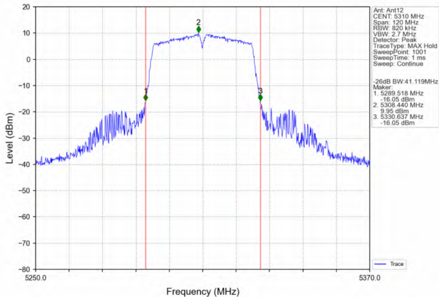
802.11n(HT40)_HCH_5310MHz_Ant12_NTNV
